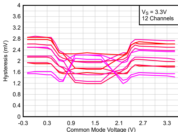
图 5-10. 迟滞与 共模电压间的关系, 3.3V
