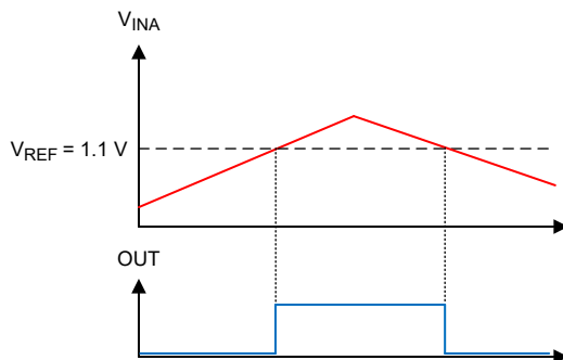
图 7-8. 过流结果
