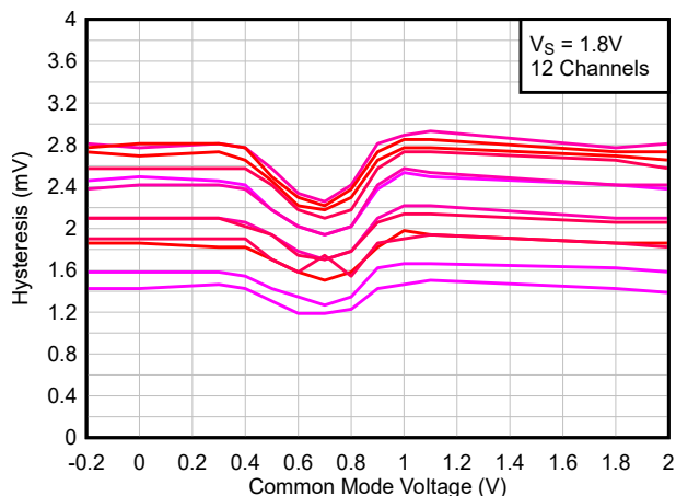
图 5-8. 迟滞与 共模电压间的关系, 1.8V
