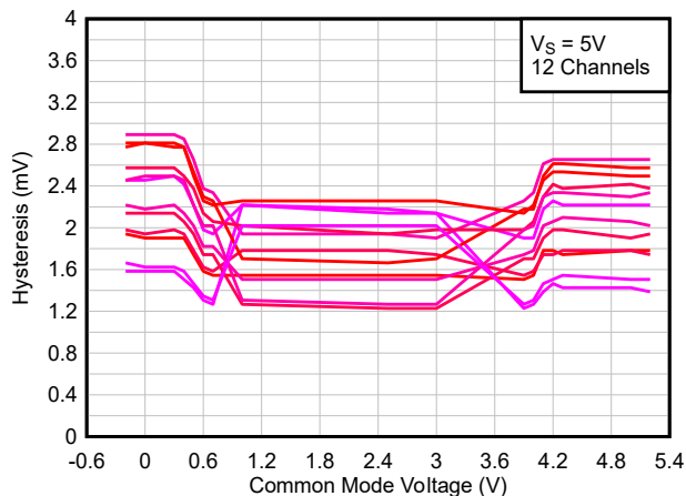
图 5-12. 迟滞与 共模电压间的关系, 5V
