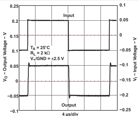
图 5-27. 小信号同相应
