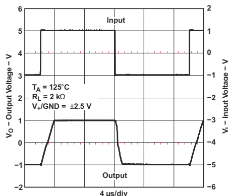
图 5-30. 大信号同相应
