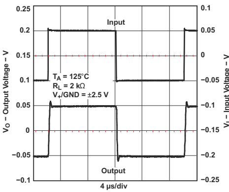
图 5-29. 小信号同相应
