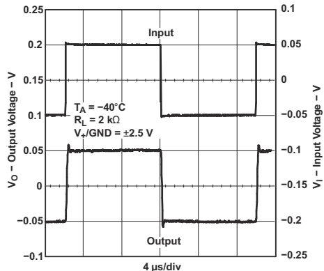
图 5-25. 小信号同相应
