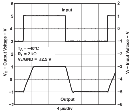
图 5-26. 大信号同相应
