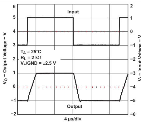
图 5-28. 大信号同相应
