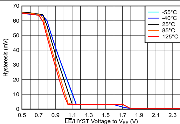
图 5-38. 迟滞电压与 \overline{\text{LE}}/\text{HYST} 电压间的关系, 5\text{V}
