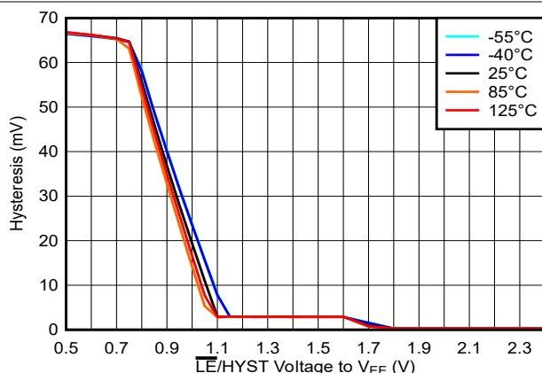
图 5-36. 迟滞电压与 \overline{\text{LE}}/\text{HYST} 电压间的关系, 2.5\text{V}
