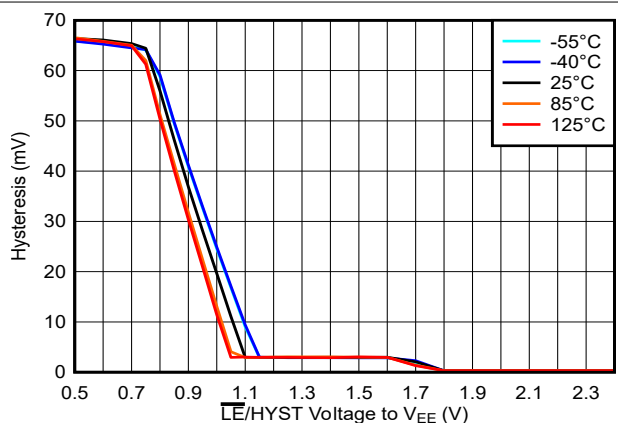
图 5-37. 迟滞电压与 \overline{\text{LE}}/\text{HYST} 电压间的关系, 3.3\text{V}
