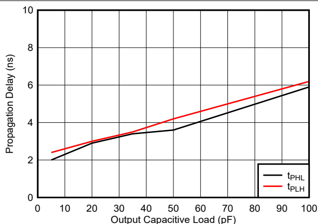
图 5-33. 传播延迟与负载电容间的关系, 3.3\text{V}
