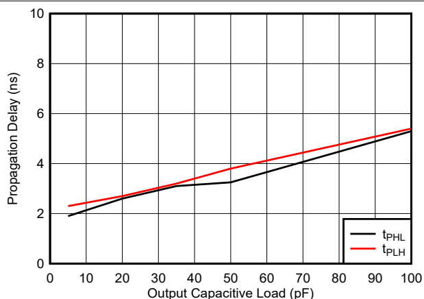
图 5-34. 传播延迟与负载电容间的关系, 5\text{V}
