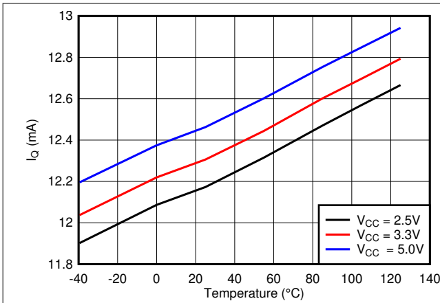
图 5-1. I_Q vs Temperature
