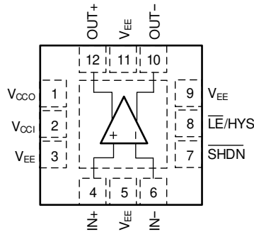
图 4-2. RVK Package 12-Pin QFN Top View
