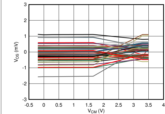
图 5-3. V_{OS} vs V_{CM} @ V_{CC} = 3.3\text{V} - 50 Devices
