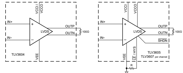
功能方框图
