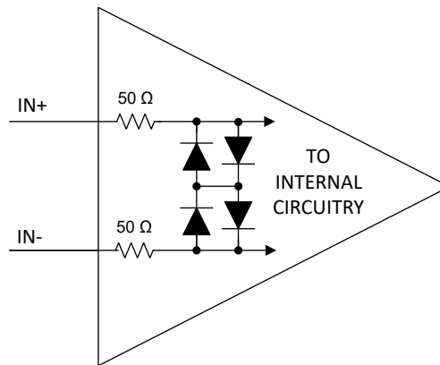
图 7-1. Input Stage Circuitry
