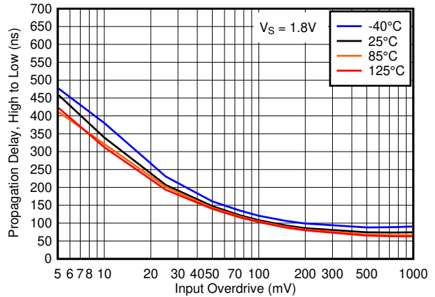
图 6-14. 传播延迟, 从高电平到低电平, 1.8V
