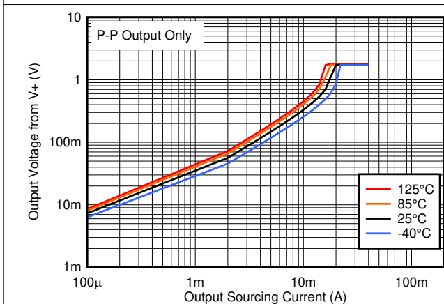
图 6-5. 输出拉电流与输出电压间的关系，1.8V
