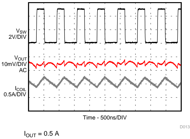
图 14. PWM Operation
