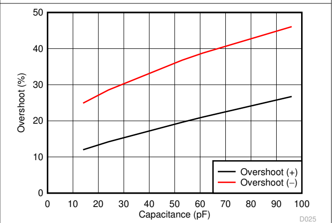
图 7-26. 小信号过冲与负载电容间的关系
