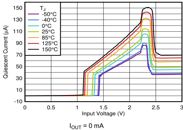
图 6-9. I_Q Increase Below Minimum V_{IN}
