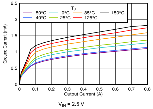
图 6-8. I_{GND} vs I_{OUT}
