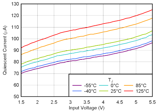
图 5-7. 静态电流与 V_{IN} 间的关系
