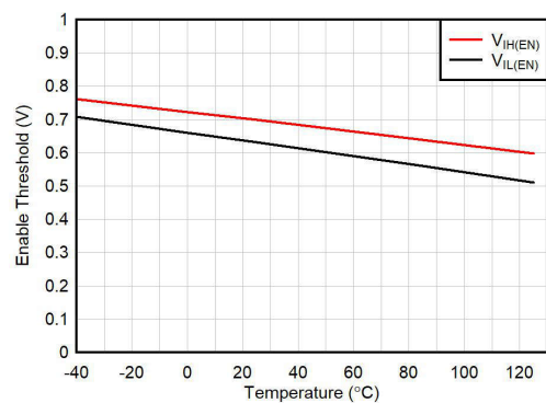
图 5-12. 使能逻辑阈值与温度间的关系
