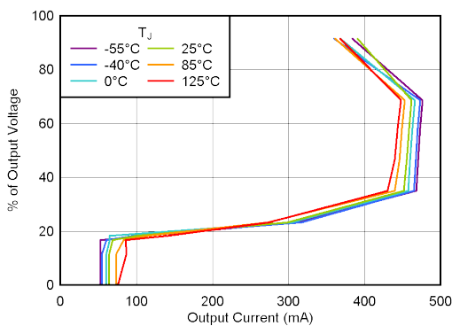
图 5-11. 电流限值
