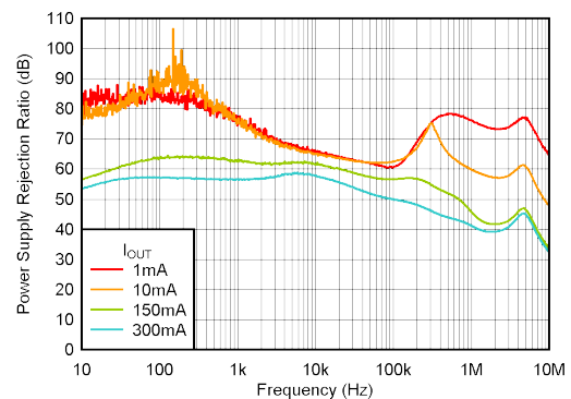
图 7-3. PSRR
