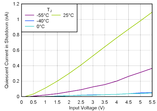
图 5-10. 关断电流与 V_{IN} 间的关系
