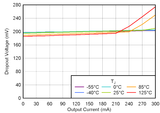
图 5-6. 压降与 I_{OUT} 间的关系
