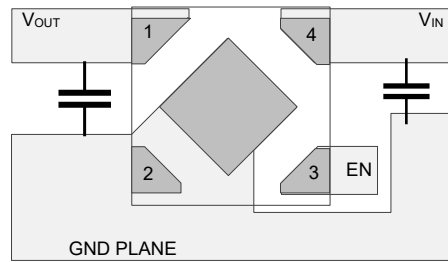
图 7-4. DQN 封装 (X2SON) 典型布局
