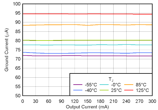
图 5-8. 接地电流与 I_{OUT} 间的关系
