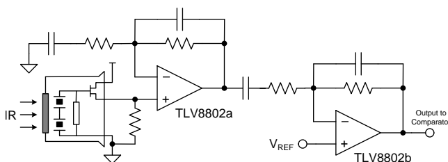
毫微功耗 PIR 运动传感器放大器
