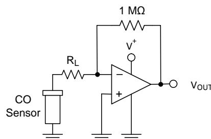
毫微功耗 CO 传感器
