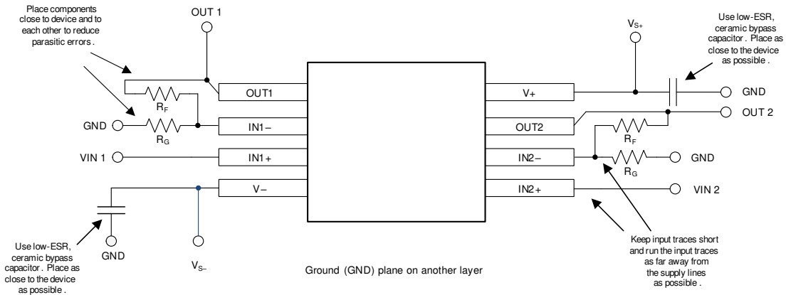
图 9-8. 布局示例
