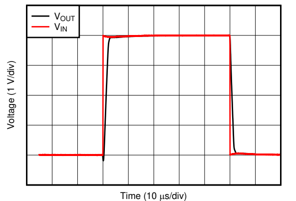
图 7-28. 过载恢复
