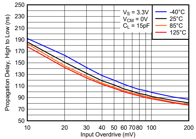
图 5-26. 传播延迟, 从高电平到低电平, 3.3V
