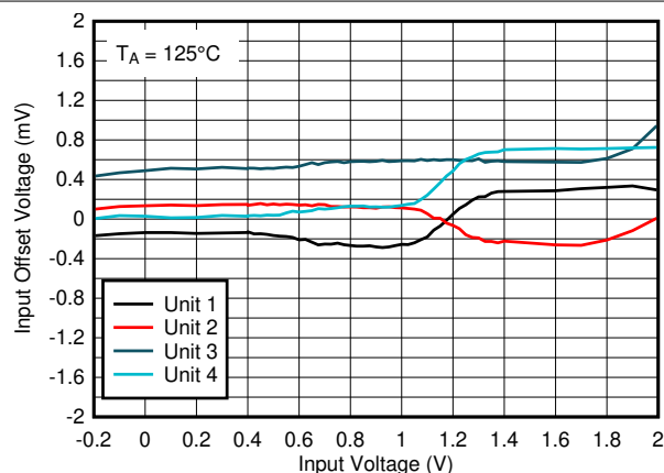
图 5-23. 125^\circ\text{C} 时失调电压与输入电压间的关系, 1.8V
