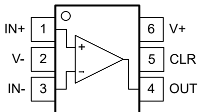
图 4-1. DCK 和 DBV 封装 标准 东 引脚排列 6 引脚 SC-70 和 SOT-23 顶视图
