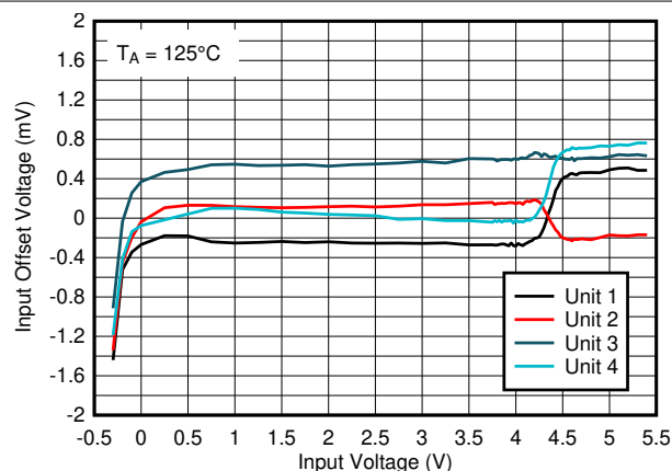
图 5-24. 125^\circ\text{C} 时失调电压与输入电压间的关系, 5V
