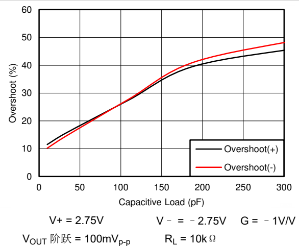
图 8-24. 小信号过冲与负载电容间的关系
