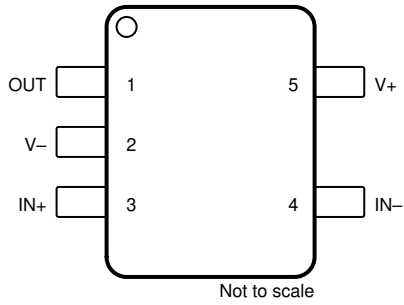
图 4-1. TLV9104-Q1 (1) DBV 封装 5 引脚 SOT-23 顶视图
