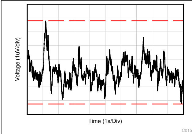
图 5-21. 0.1Hz 至 10Hz 噪声
