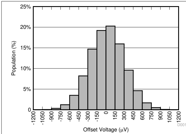
图 5-1. 失调电压产生分布
