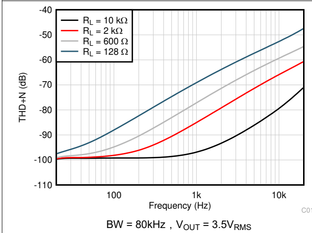
图 5-23. THD+N 比与频率间的关系
