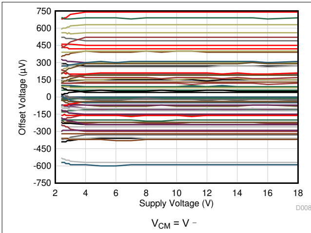
图 5-9. 失调电压与电源间的关系 每种颜色代表一个样本器件。
