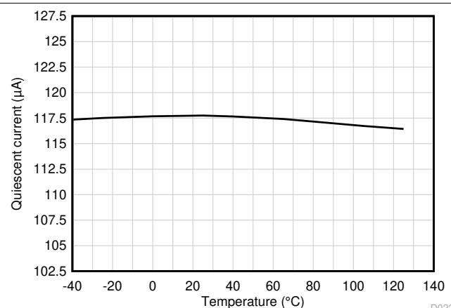
图 5-26. 每通道静态电流与温度间的关系
