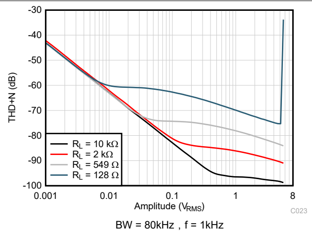
图 5-24. THD+N 与输出幅度间的关系
