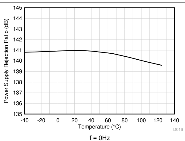
图 5-20. PSRR 与温度间的关系 (dB)
