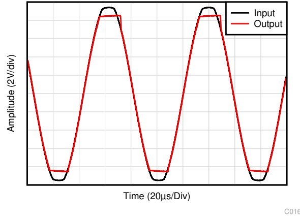
图 6-2. 无相位反转
