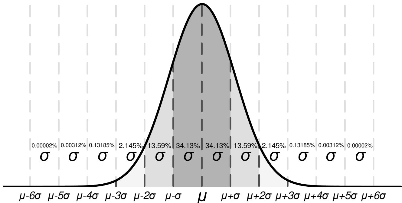
图 6-9. 高斯分布
