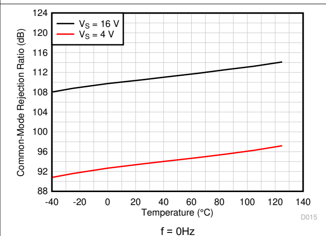
图 5-19. CMRR 与温度间的关系 (dB)
