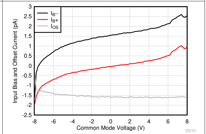
图 5-12. 输入偏置电流与共模电压间的关系
