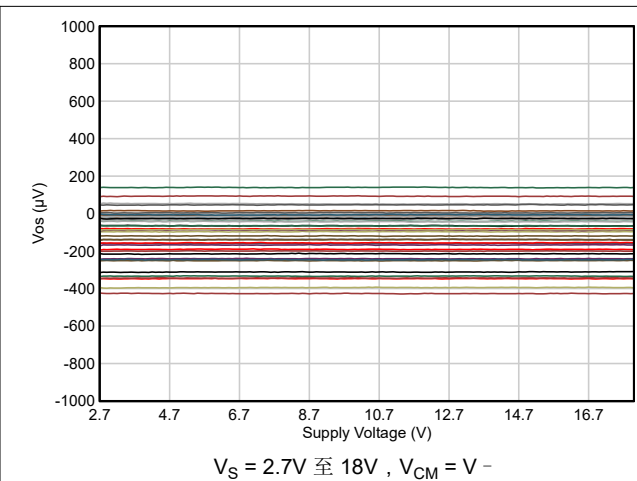
图 5-20. 输入失调电压与电源电压间的关系
