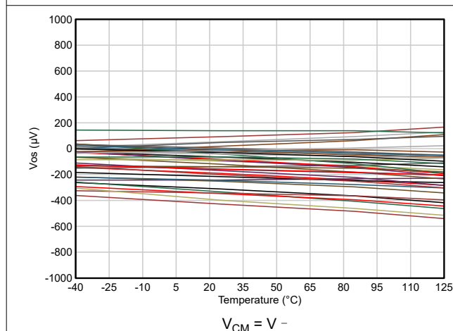
图 5-15. 输入失调电压与温度间的关系
