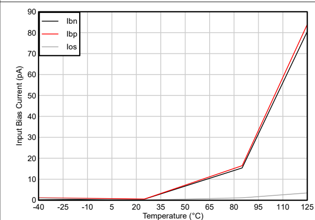
图 5-22. 输入偏置电流与温度间的关系
