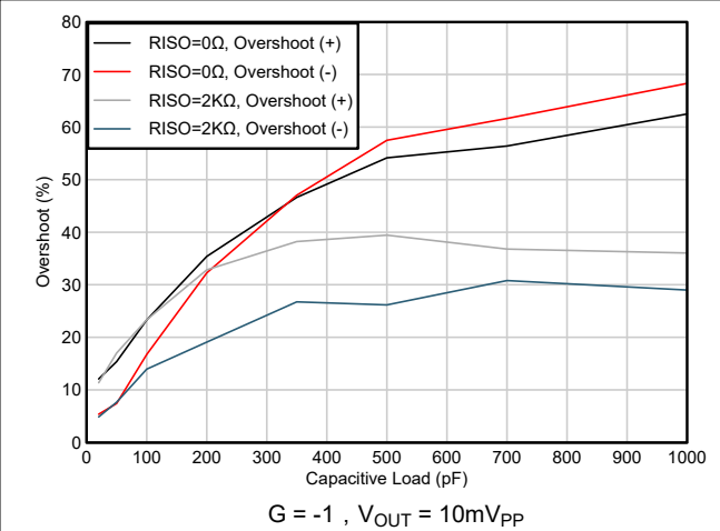
图 5-34. 小信号过冲与容性负载间的关系
