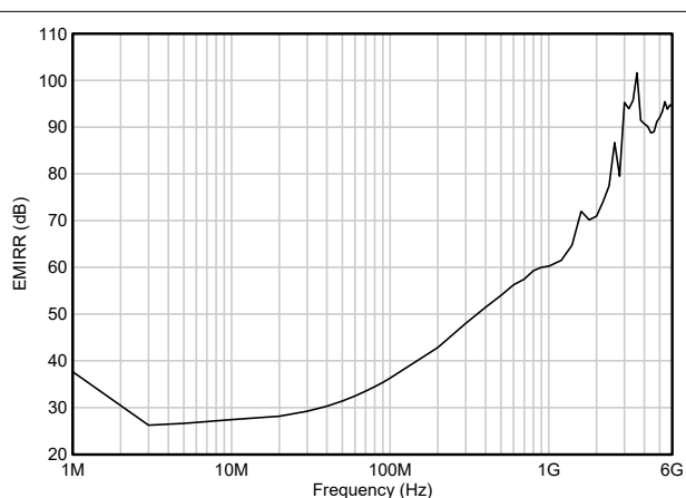
图 5-14. EMIRR 与频率间的关系
