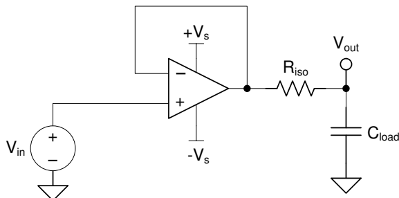
图 6-5. 使用 TLV9151-Q1 扩展容性负载驱动
