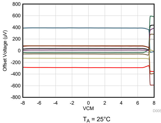
图 5-5. 失调电压与共模电压间的关系
