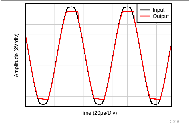
图 6-29. 无相位反转
