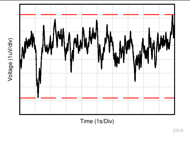
图 5-18. 0.1Hz 至 10Hz 噪声
