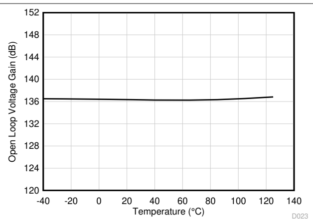
图 5-24. 开环电压增益与温度间的关系 (dB)
