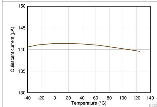
图 5-23. 静态电流与温度间的关系
