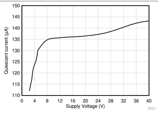
图 5-22. 静态电流与电源电压间的关系
