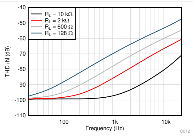
图 5-20. THD+N 比与频率间的关系
