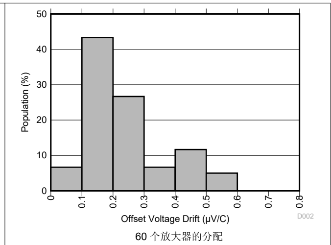
图 5-2. 失调电压漂移分配
