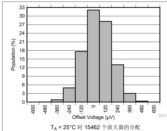
图 5-1. 失调电压生产分配
