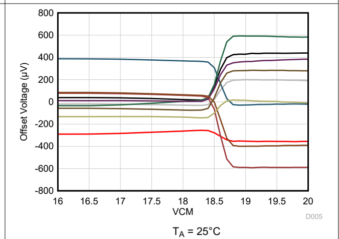
图 5-6. 失调电压与共模电压间的关系 (切换区域)
