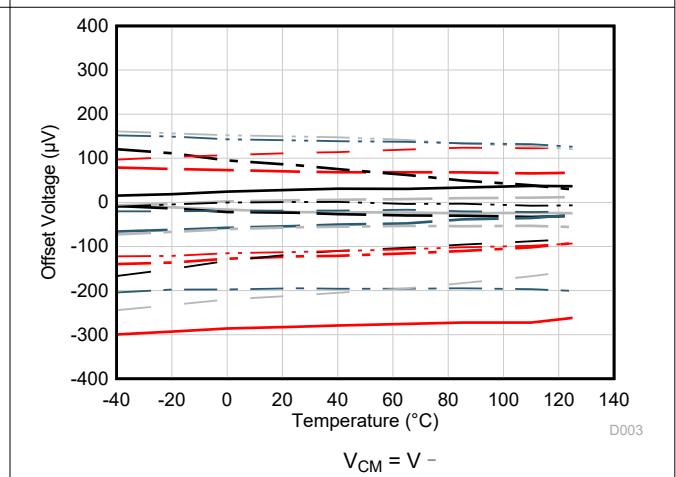
图 5-4. 失调电压与温度间的关系
