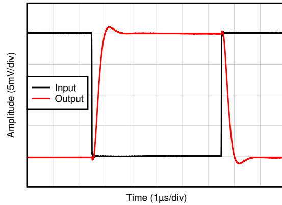
图 5-32. 负过载恢复
