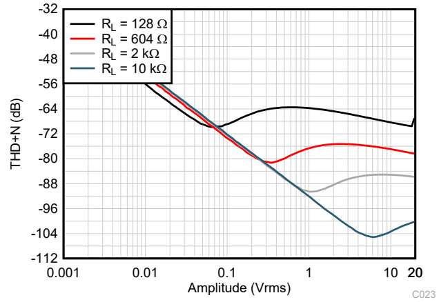
图 5-22. THD+N 与输出幅度间的关系
