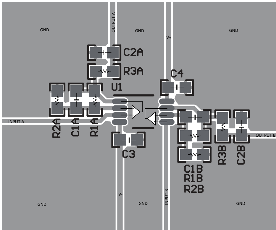
图 7-6. VSSOP-8 (DGK) 封装的布局示例
