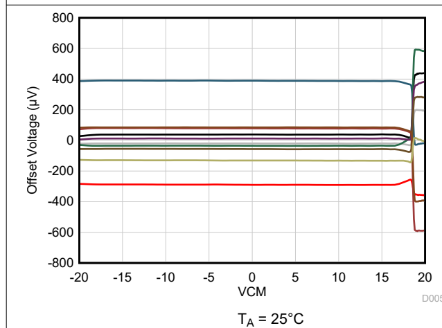
图 5-5. 失调电压与共模电压间的关系
