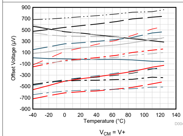
图 5-3. 失调电压与温度之间的关系
