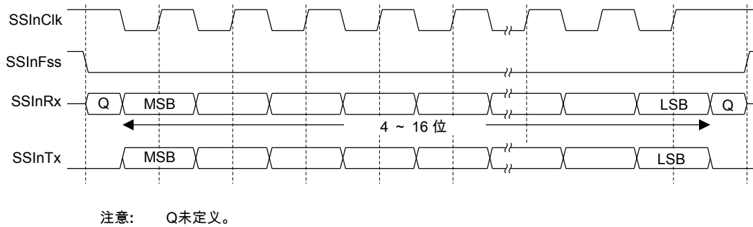
图 15-9. SPO = 1、SPH = 1 时的飞思卡尔 SSI 帧格式
