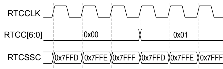
图 7-6. TRIM 值为 0x7FFC 时的计数器行为
