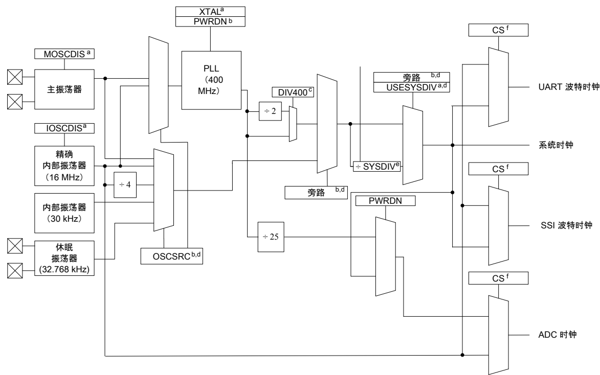
图 5-5. 主时钟树
