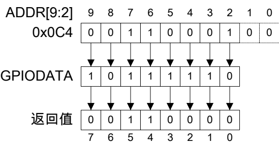
图 10-4. GPIODATA 读实例
