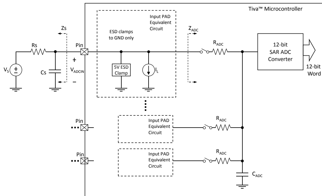
图 21-19. ADC Input Equivalency Diagram
