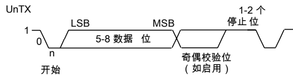
图 14-2. UART字符帧
