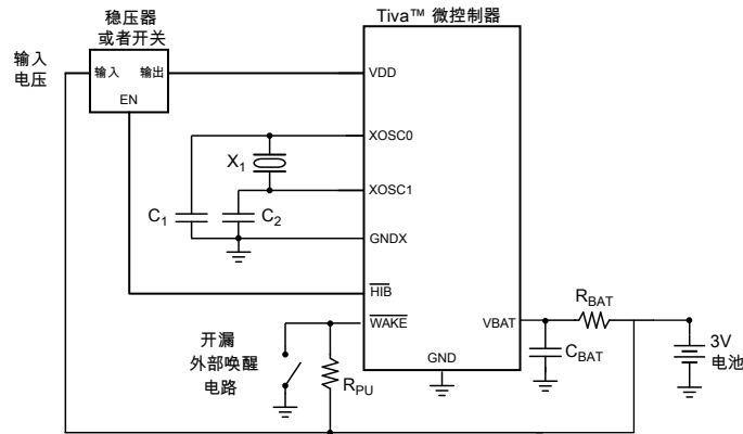
图 7-2. 使用晶振作为睡眠模块的时钟源 ( 单一电池源 )
