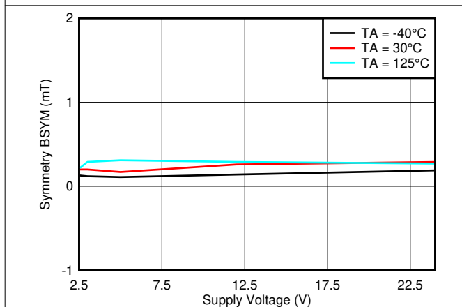
图 6-23. B_{SYM(Y)} 与 V_{CC} 间的关系
