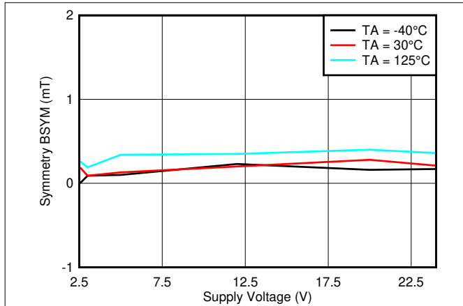
图 6-19. B_{SYM(Z)} 与 V_{CC} 间的关系
