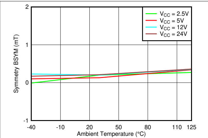
图 6-20. B_{SYM(Z)} 与温度间的关系
