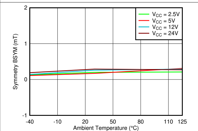
图 6-24. B_{SYM(Y)} 与温度间的关系
