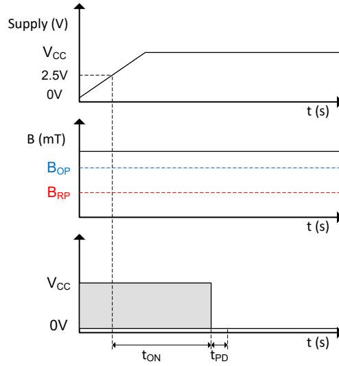
图 7-20. B > B_{OP} 时的上电时间 (R 引脚排列版本)
