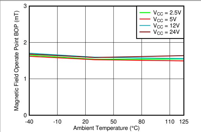
图 6-14. BOP_Y 阈值与温度间的关系
