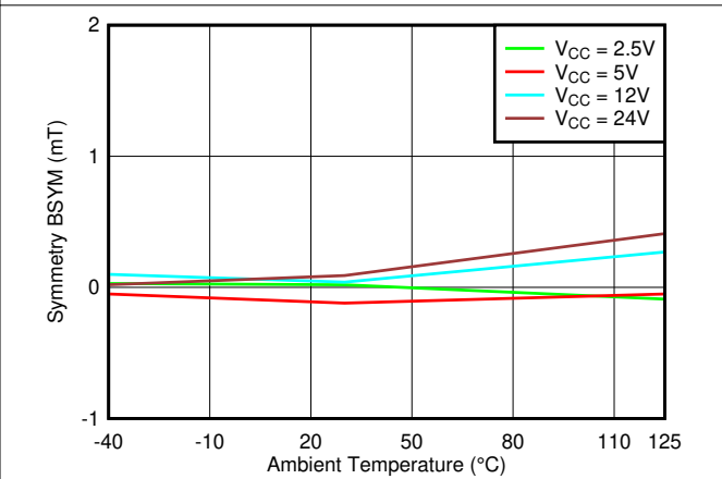
图 6-22. B_{SYM(X)} 与温度间的关系
