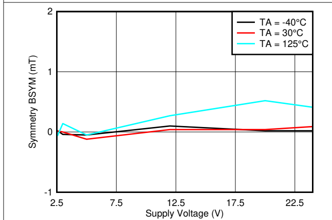
图 6-21. B_{SYM(X)} 与 V_{CC} 间的关系
