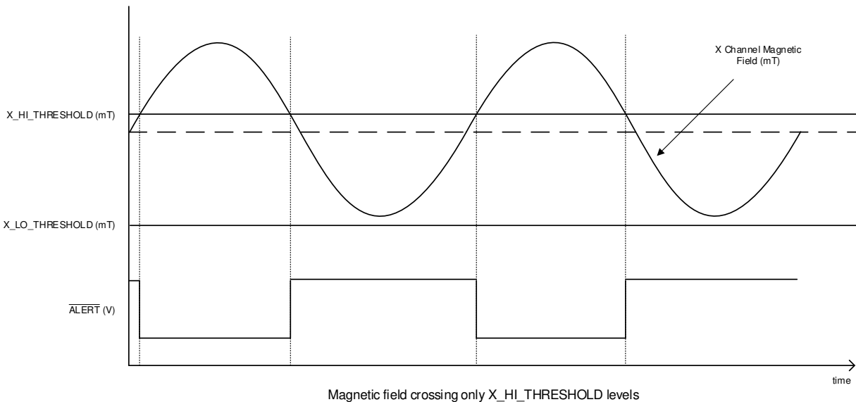
图 7-3. ALERT 引脚用作磁性开关
