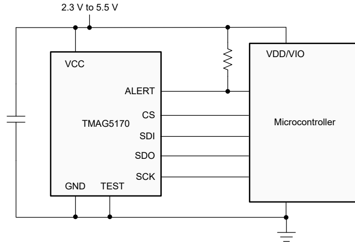
图 7-4. TMAG5170D-Q1 Application Diagram
