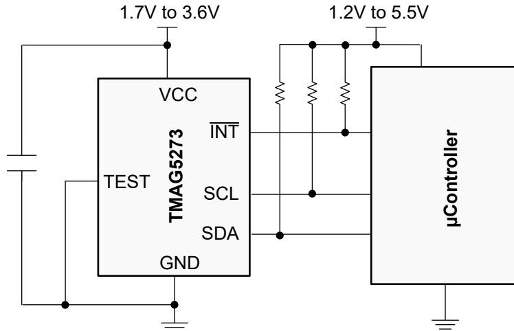
应用方框图
