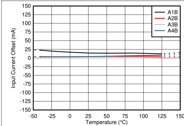
图 7-3. TMCS1101AxB 输入失调电流与温度间的关系
