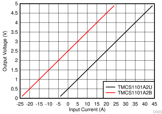
图 9-14. TMCS1101A2B 和 TMCS1101A2U
