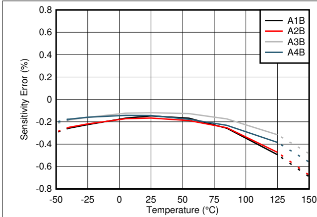
图 7-1. TMCS1101AxB 灵敏度误差与温度间的关系
