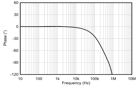
图 6-12. 相位与频率间的关系 (所有增益)
