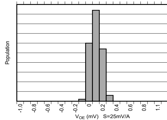
图 6-6. 失调误差产生分布图
