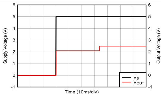
图 6-19. 启动瞬态响应
