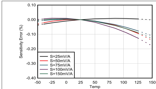
图 6-1. 灵敏度误差与温度间的关系
