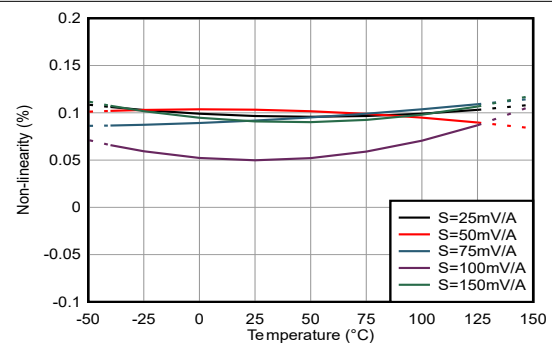
图 6-4. 非线性与温度间的关系
