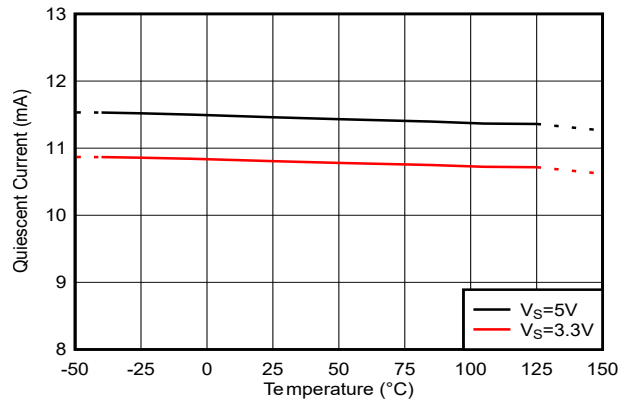
图 6-14. 静态电流与温度间的关系
