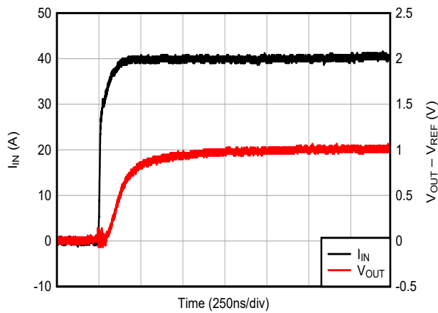
图 6-9. 电压输出阶跃响应 (上升)
