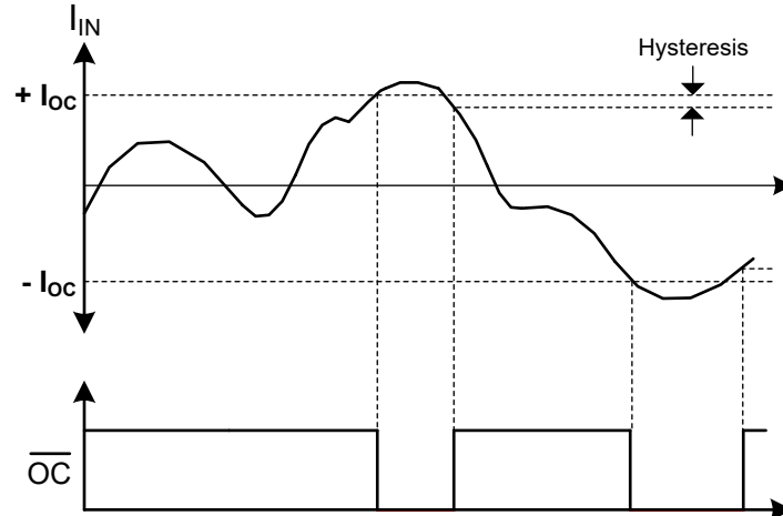
图 8-7. 过流检测图
