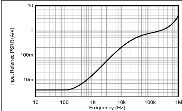
图 6-3. PSRR 与频率间的关系
