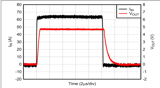
图 6-7. 电流过载响应
