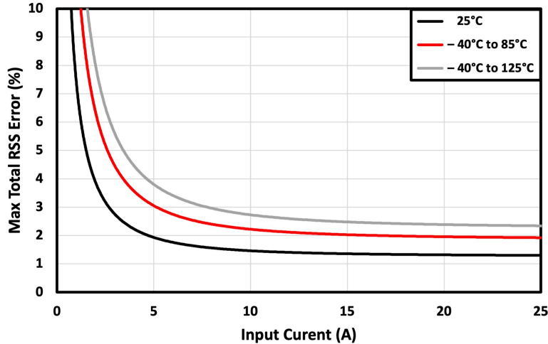
图 9-1. RSS 误差与输入电流间的关系
