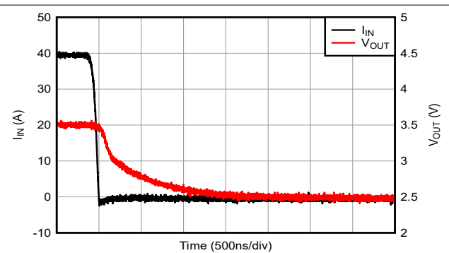
图 6-6. 电压输出阶跃响应 (下降)
