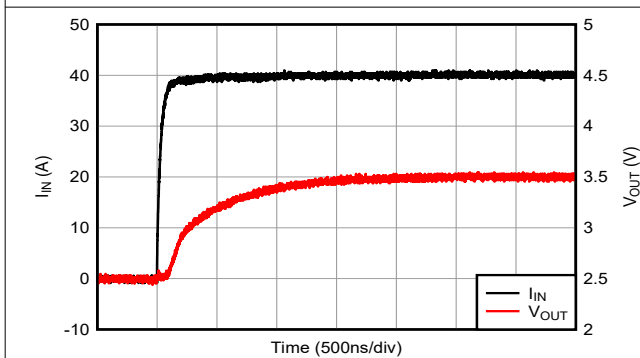
图 6-5. 电压输出阶跃响应 (上升)
