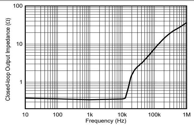
图 6-4. 输出阻抗与频率间的关系
