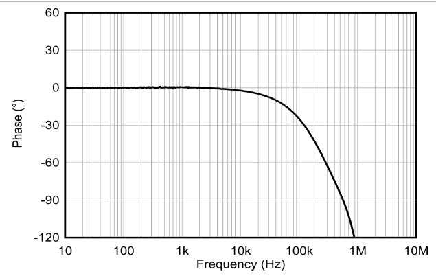
图 6-2. 相位与频率间的关系 (所有增益)
