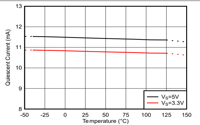
图 6-10. 静态电流与温度间的关系
