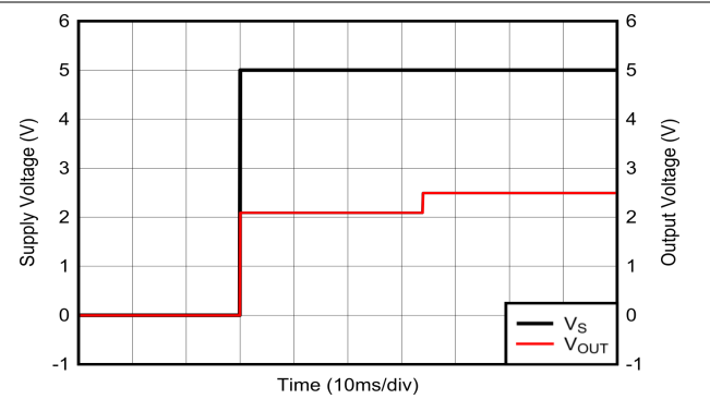
图 6-8. 启动瞬态响应
