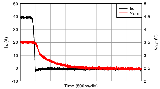
图 6-6. 电压输出阶跃响应 (下降)
