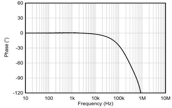
图 6-2. 相位与频率间的关系 (所有增益)
