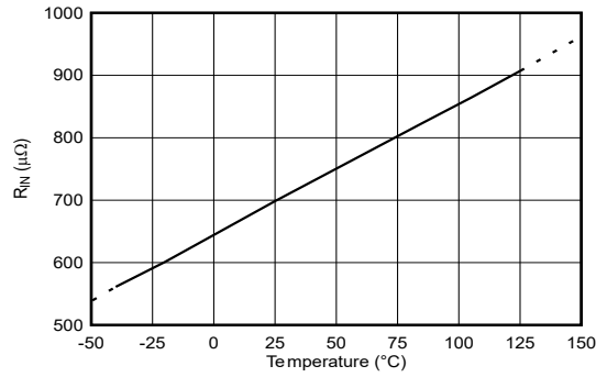
图 6-11. 输入导体电阻与温度间的关系
