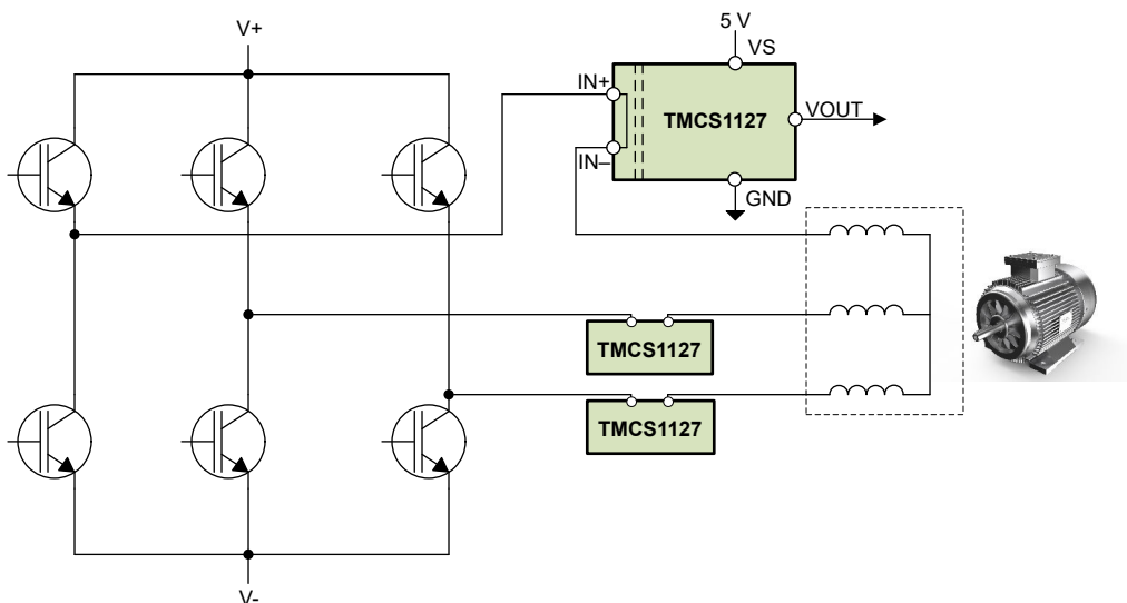
图 9-2. 内嵌式电机相电流检测
