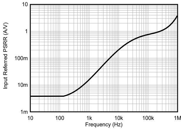
图 6-9. PSRR 与频率间的关系
