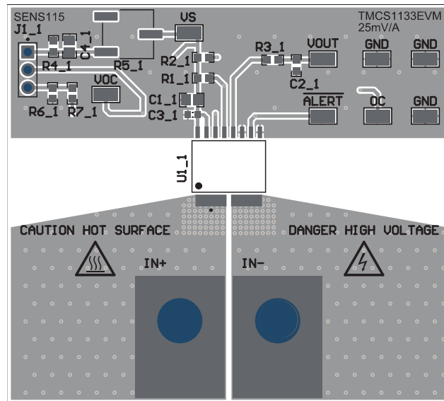
图 9-6. 建议的电路板布局布线
