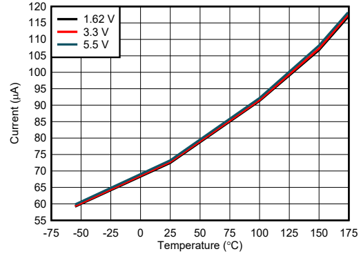
图 7-6. 有效转换电流与温度间的关系
