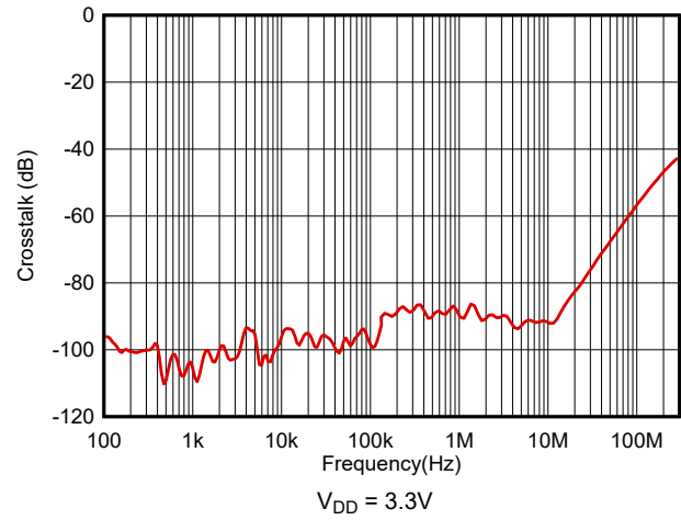
图 5-20. 串扰与频率间的关系
