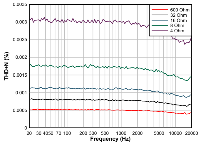
图 8-2. 不同负载条件下的 THD+N
