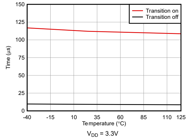
图 5-10. 转换时间与温度间的关系
