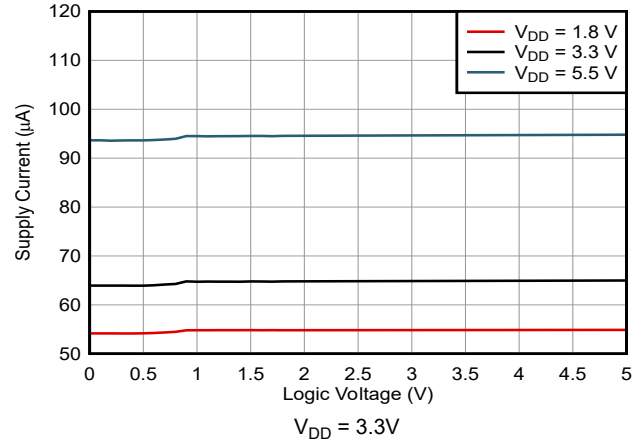
图 5-8. 电源电流与逻辑电压间的关系
