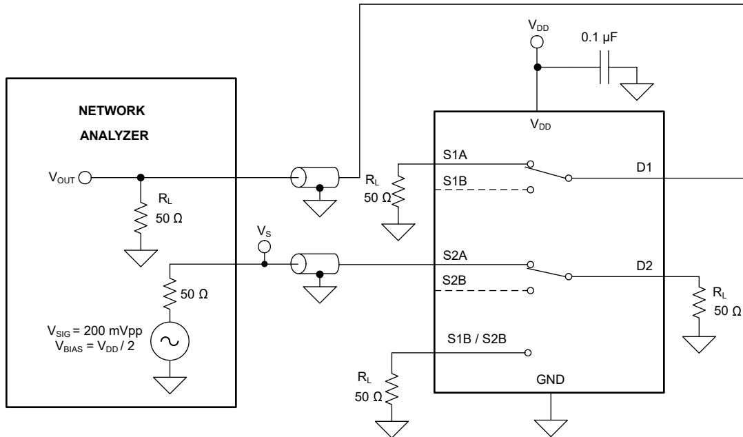
图 6-14. 串扰测量设置
