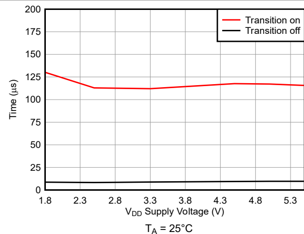
图 5-11. 转换时间与电源电压间的关系
