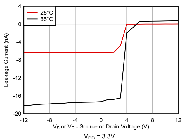
图 5-3. 导通漏电流与源极或漏极电压间的关系
