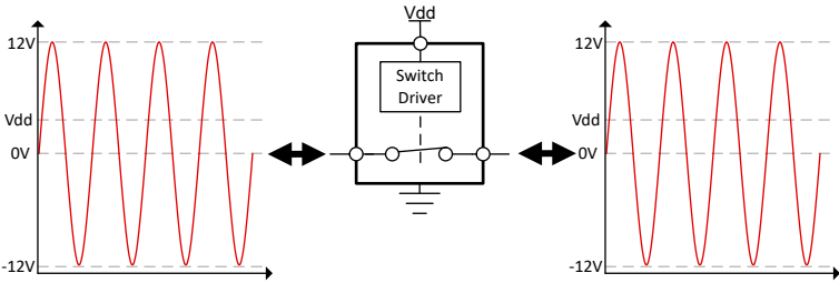
图 7-1. 支持超出电源电压的信号
