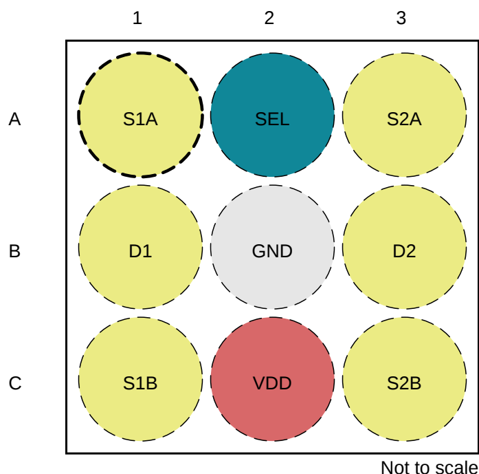
图 4-1. YBH 封装，9 焊球 DSBGA ( 顶视图，凸点面朝下 )
