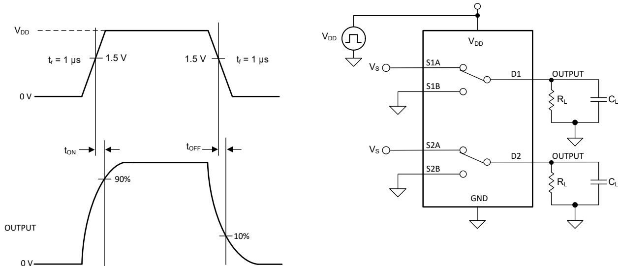
图 6-6. t_{ON}(V_{DD}) 和 t_{OFF}(V_{DD}) 时间测量设置
