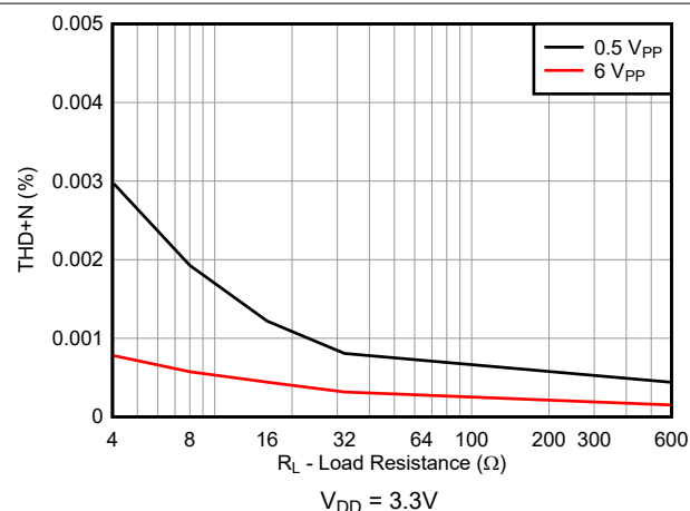
图 5-17. THD+N 与负载阻抗间的关系
