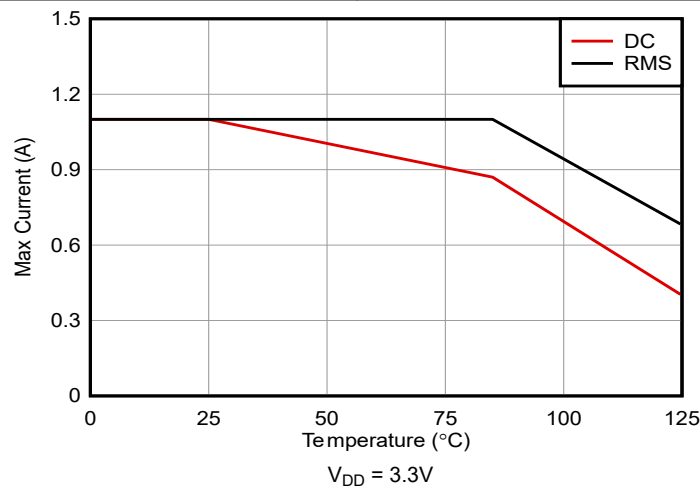
图 5-23. 最大连续电流与温度间的关系
