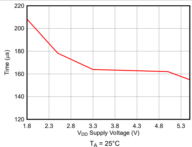
图 5-12. tBBM 与电源电压间的关系
