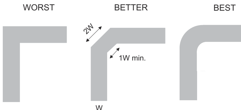
图 8-3. 布线示例
