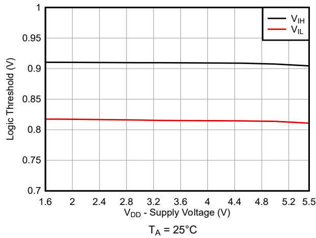
图 5-9. 逻辑阈值与电源电压间的关系
