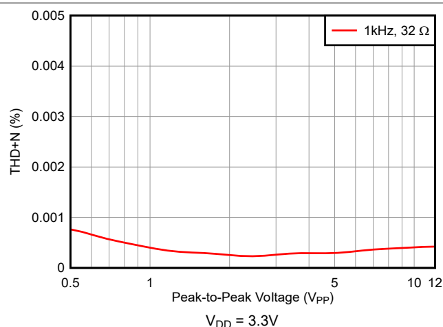
图 5-16. THD+N 与峰峰值电压间的关系
