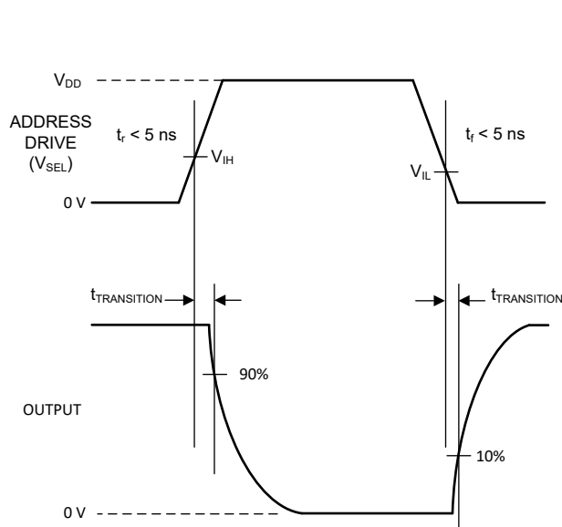
图 6-7. 转换时间测量设置
