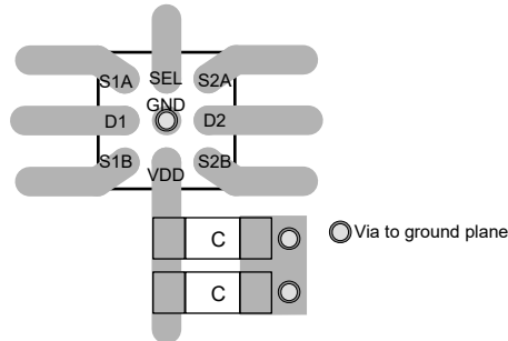
图 8-4. TMUX4827 布局示例
