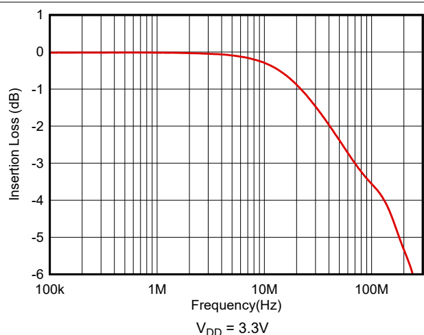
图 5-18. 插入损耗与频率间的关系
