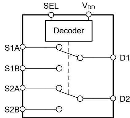
TMUX4827 方框图
