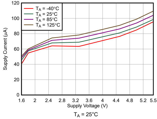
图 5-7. 电源电流与电源电压间的关系
