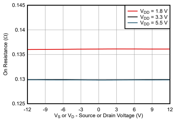
导通电阻与源极或漏极电压之间的关系
