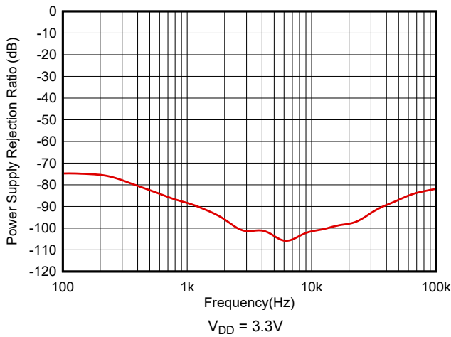
图 5-21. ACPSRR 与频率间的关系
