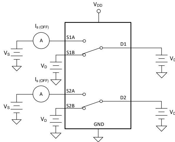
图 6-3. 关断漏电流测量设置
