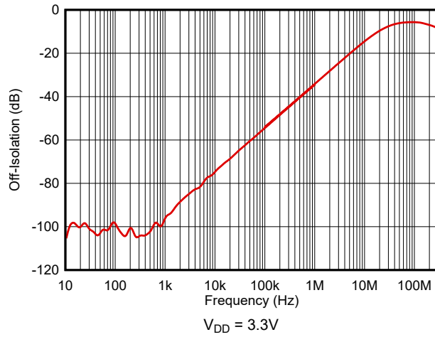
图 5-19. 关断隔离与频率间的关系
