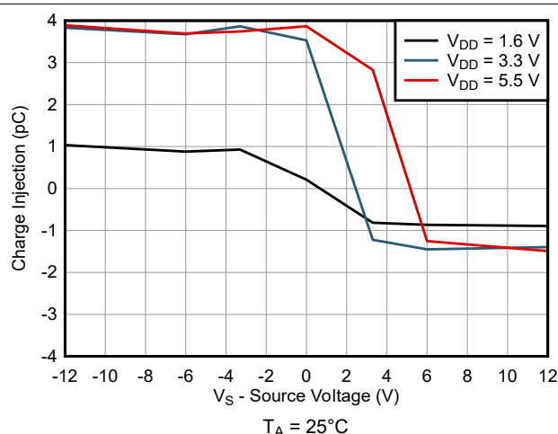
图 5-13. 电荷注入与源极电压间的关系
