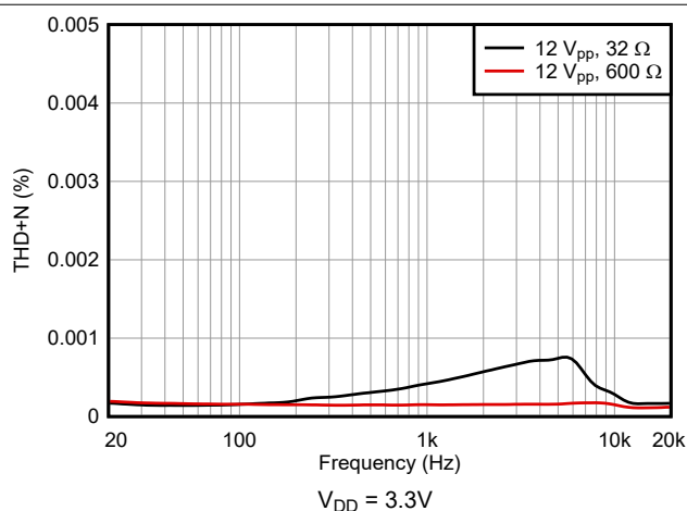
图 5-15. THD+N 与频率间的关系
