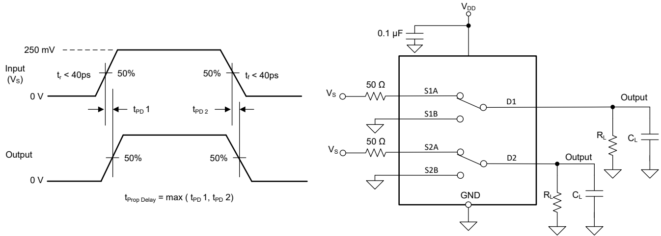
图 6-5. 传播延迟测量设置
