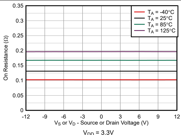
图 5-2. 导通电阻与温度间的关系
