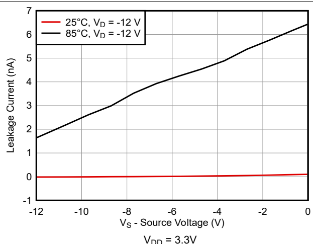
图 5-4. ISOFF 漏电流与源极电压间的关系
