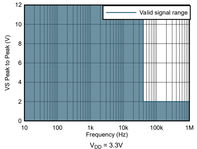
图 5-22. 最大信号摆幅
