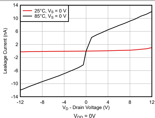
图 5-5. IDOFF 漏电流与漏极电压间的关系
