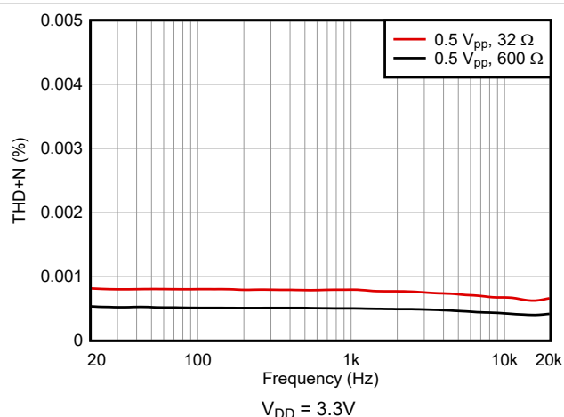
图 5-14. THD+N 与频率间的关系
