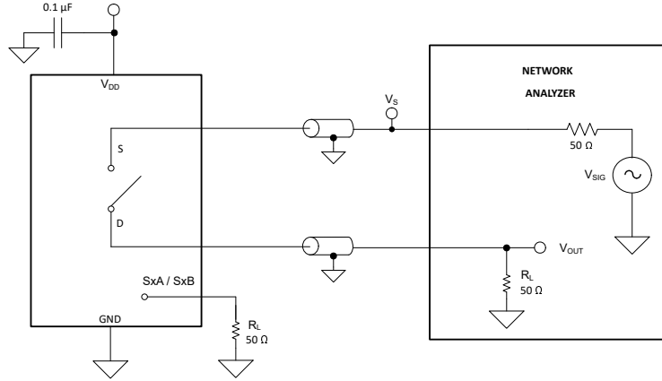
图 6-13. 关断隔离测量设置
