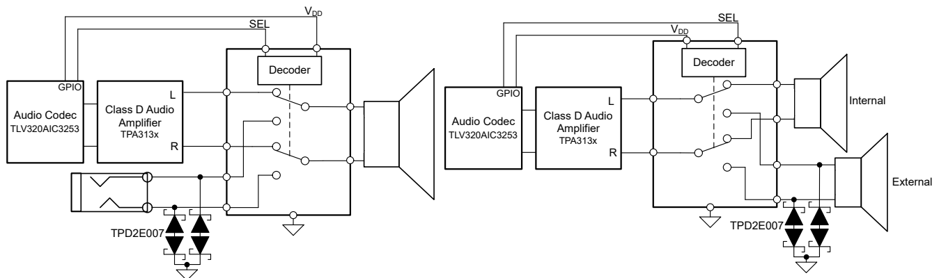
图 8-1. 音频放大器切换
