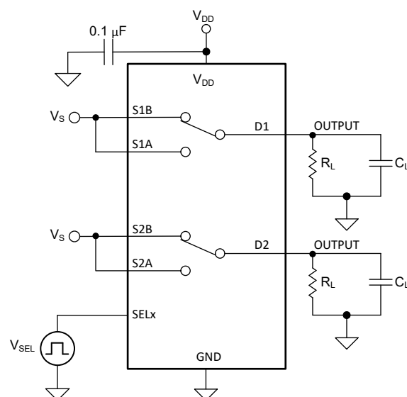
图 6-8. 先断后合延迟测量设置
