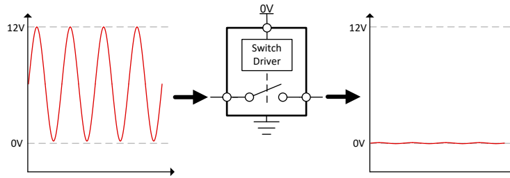
图 7-2. 支持超出电源电压的信号
