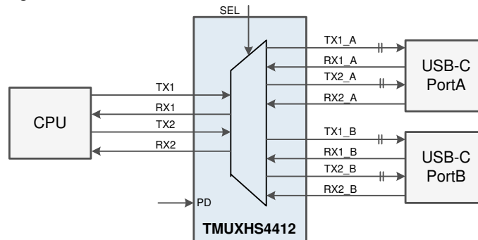
图 7-10. USB 4.0 / TBT 3.0 Demuxing
