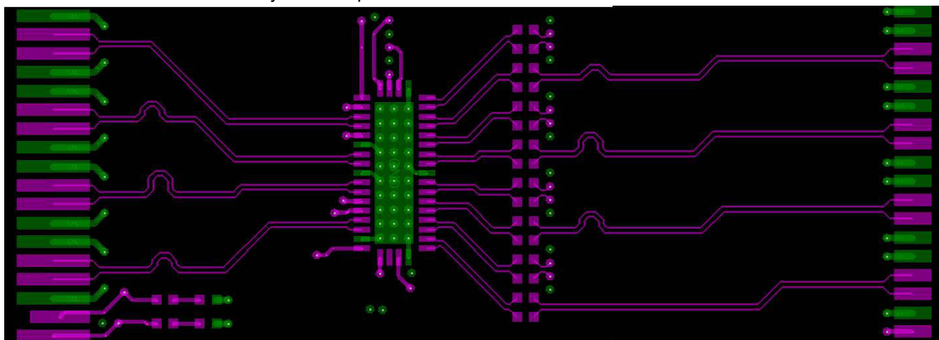
图 7-11. TMUXHS4412 Layout Example
