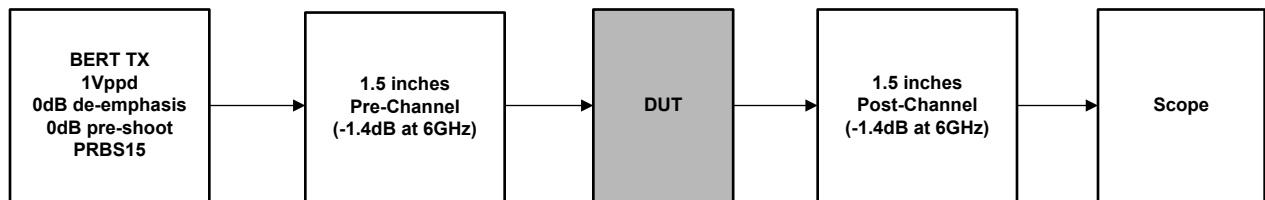
图 8-3. 测试设置
