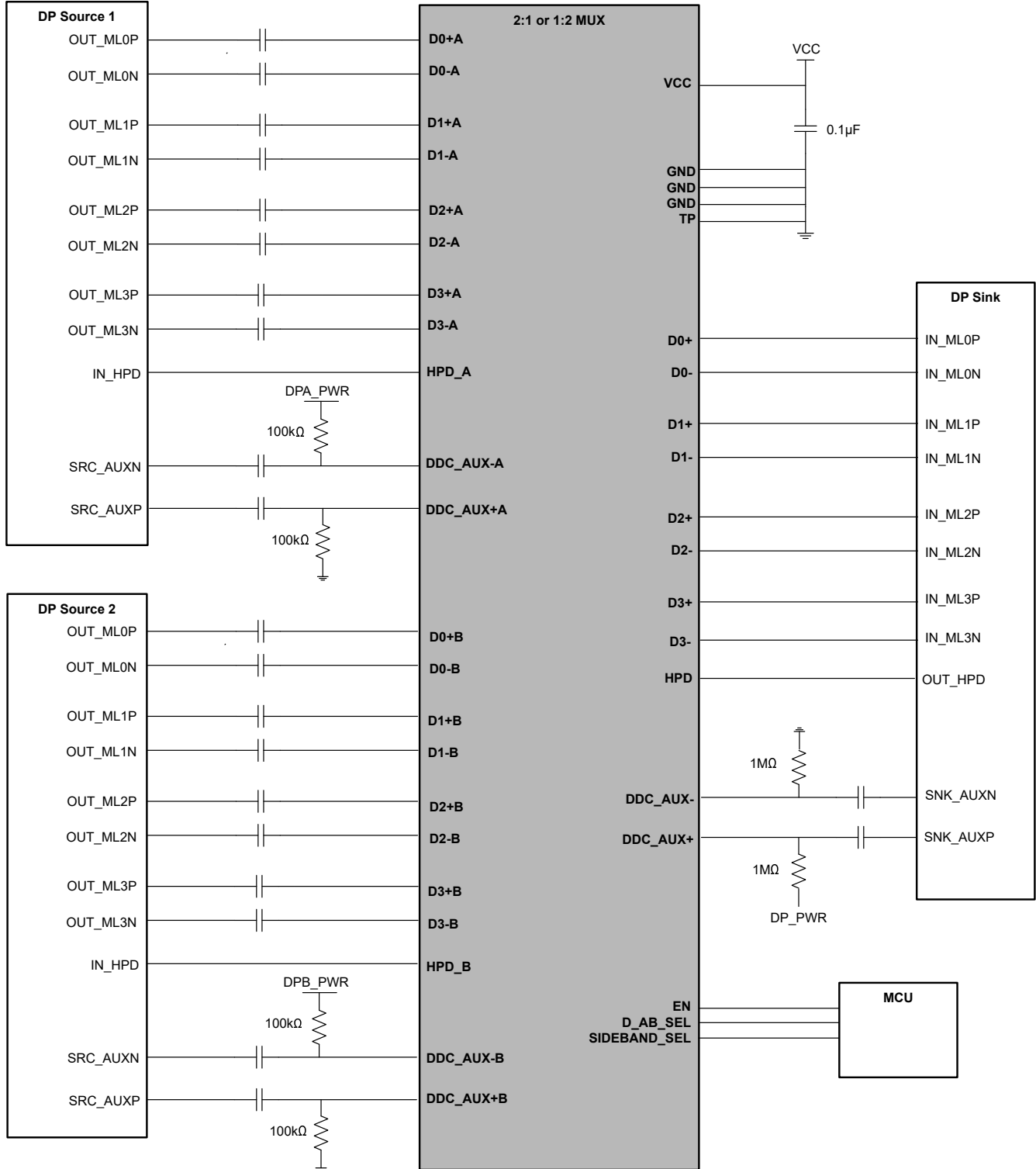
图 8-7. DisplayPort 2:1 开关
