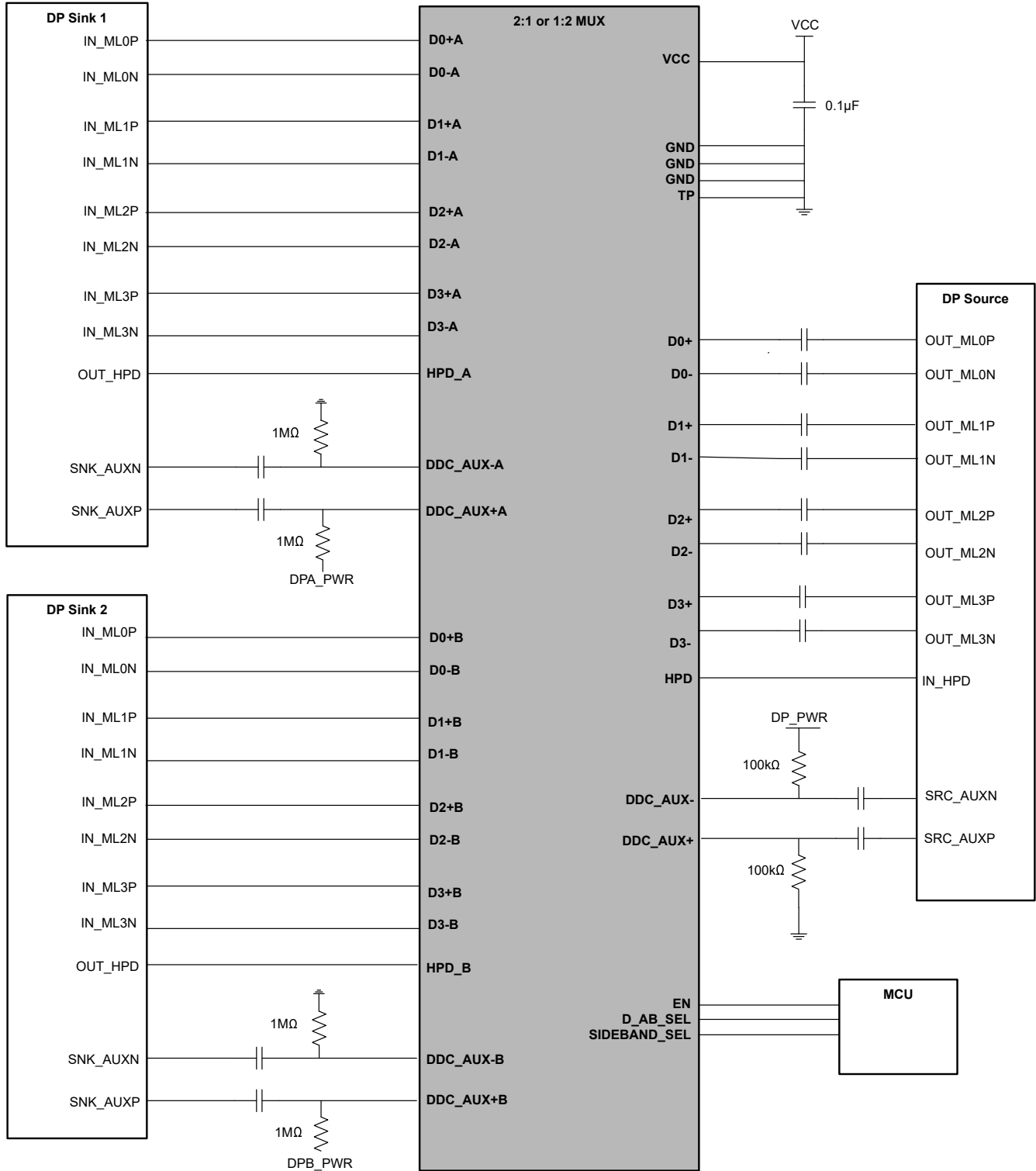
图 8-8. DisplayPort 1:2 开关
