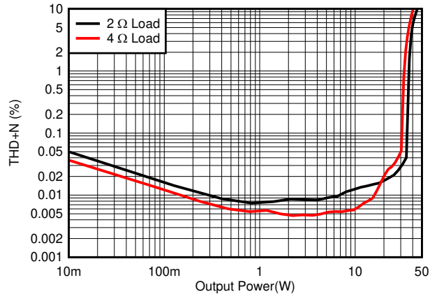
图 6-2. THD+N vs Power - 2 Ω, 4 Ω - 18 V
