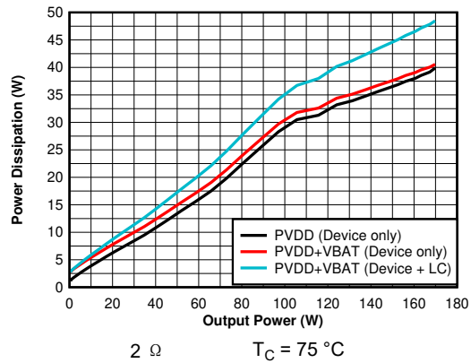
图 6-10. Power Dissipation vs Output Power - 2 \Omega
