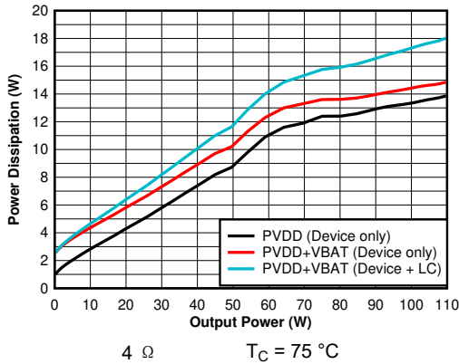
图 6-7. Power Dissipation vs Output Power - 4 \Omega
