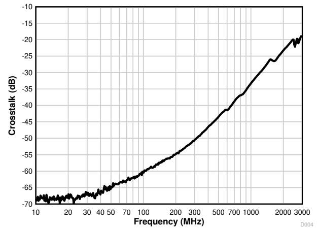
图 7-2. SBU Crosstalk
