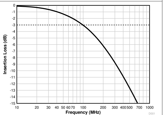
图 7-16. CC Bandwidth
