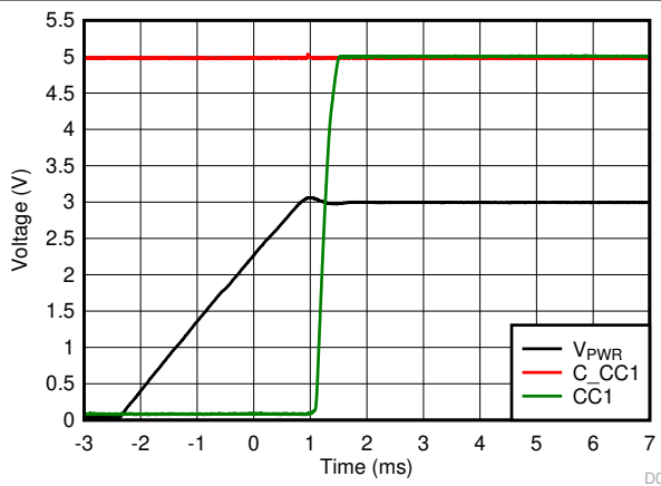
图 7-27. CC FET Turnon Timing
