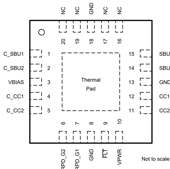
图 4-1. TPD4S481-Q1 RGR 封装，20 引脚 QFN
