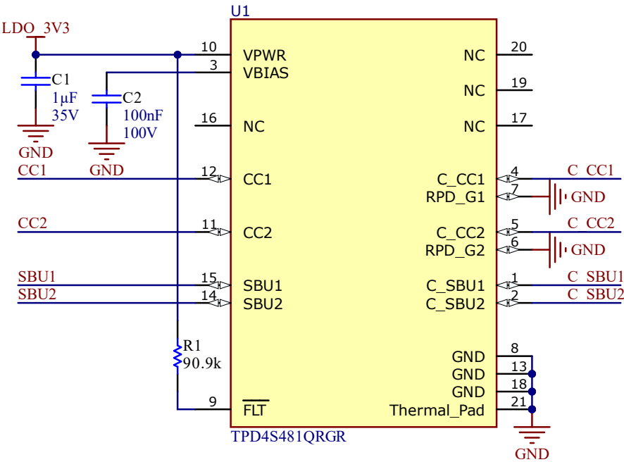
图 7-1. TPD4S481-Q1 非电池无电
