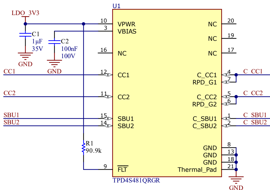
图 7-2. TPD4S481-Q1 电池无电
