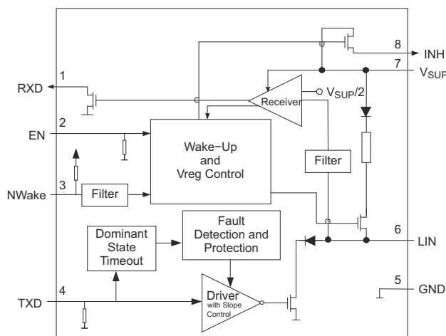
功能方框图
