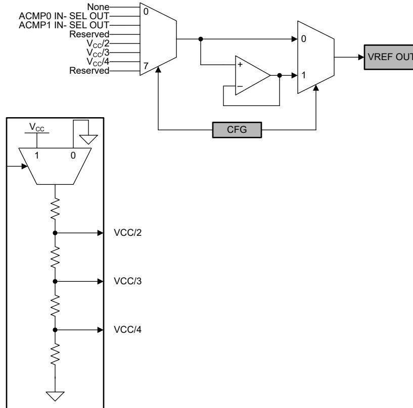
图 7-20. 电压基准方框图
