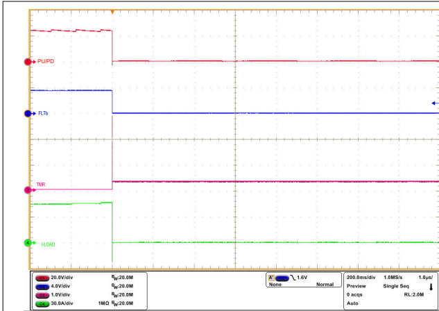
图 8-8. TPS1200-Q1 针对过流故障的闭锁响应
