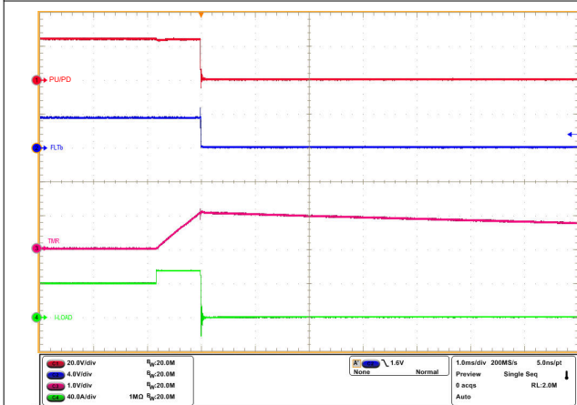
图 8-6. TPS1200-Q1 在 50A 过流保护设置且 t_{sc} = 1\text{ms} 下针对 40A 至 55A 负载阶跃的过流响应
