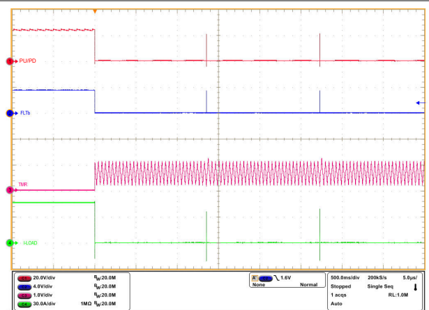
图 8-7. TPS1200-Q1 针对过流故障的自动重试响应
