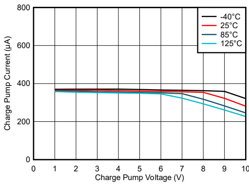
图 5-3. 电荷泵电流与电荷泵电压间的关系
