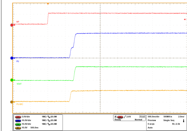
图 8-4. INP 由低电平到高电平且 C_{BST} = 470\text{nF} 时 TPS1200-Q1 的导通响应
