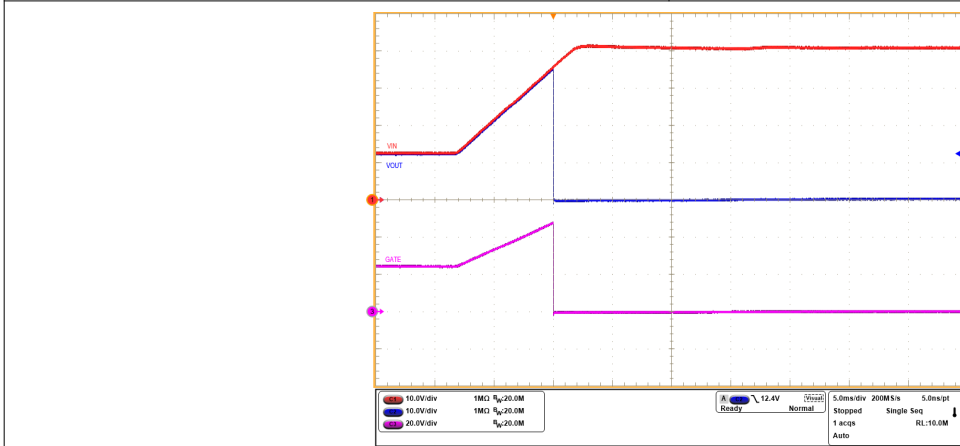
图 8-10. TPS1200-Q1 在 36V 电平下的过压截止响应
