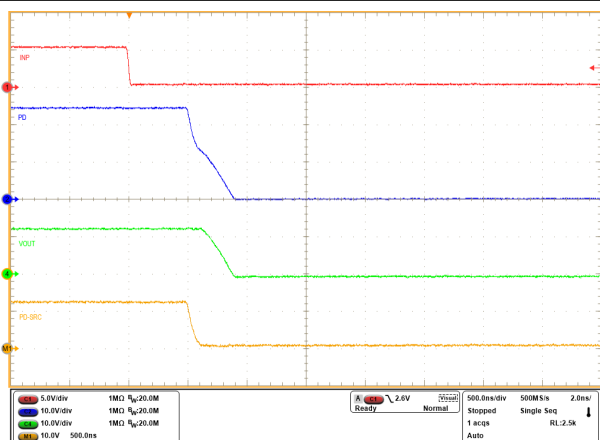
图 8-5. INP 由高电平到低电平且 C_{BST} = 470\text{nF} 时 TPS12000-Q1 的关断响应
