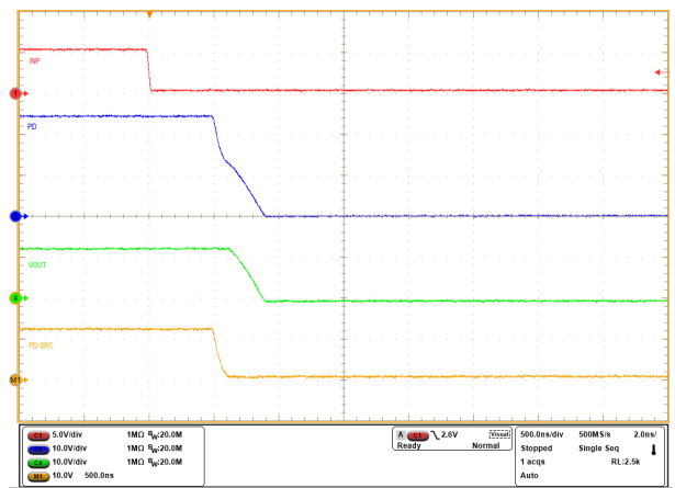
图 8-5. INP 由高电平到低电平且 C_{BST} = 470\text{nF} 时 TPS1200-Q1 的关断响应
