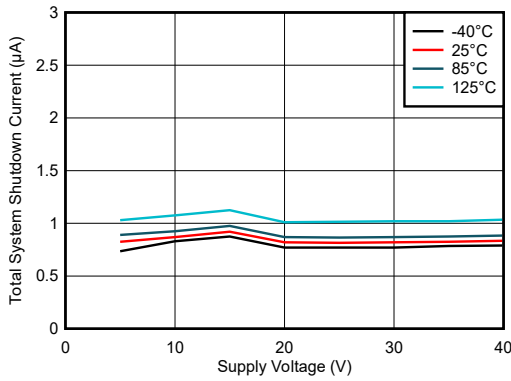
图 5-1. 关断电源电流与电源电压间的关系
