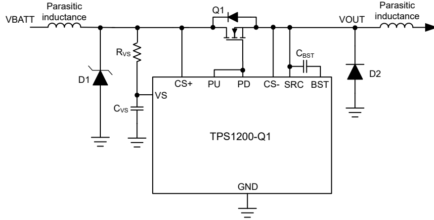
图 8-11. 采用可选保护元件的 TPS1200-Q1 电路实施方案
