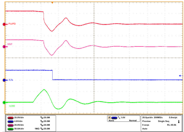
图 8-9. TPS1200-Q1 器件在 50A 短路保护设置且 TMR 为开路时的输出短路响应
