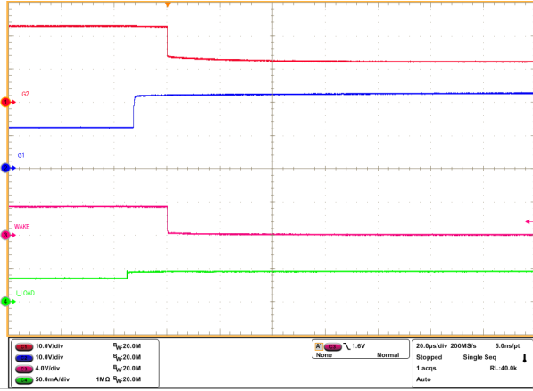
图 8-4. 从 LPM 到工作模式的状态转换放大视图 ( LPM = 低电平, VIN = 12V, EN/UVLO = 高电平 )
