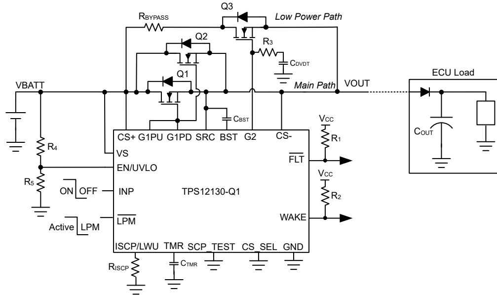
图 8-12. 适用于使用自动负载唤醒和输出大容量电容器充电功能来驱动全时供电 (PAAT) 负载的 TPS1213-Q1 应用电路
