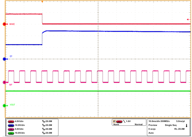
图 8-5. 由于 LPM = 低电平, 即使在唤醒后, INP 也无法控制 G1
