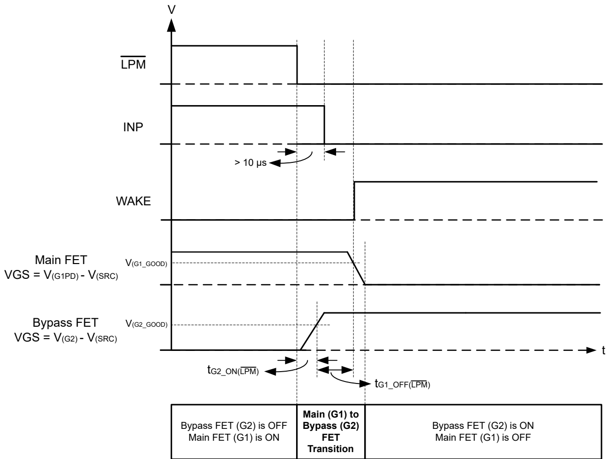
图 7-15. 从工作模式进入低功耗模式的 \overline{LPM} 和 INP 信号时序控制注意事项
