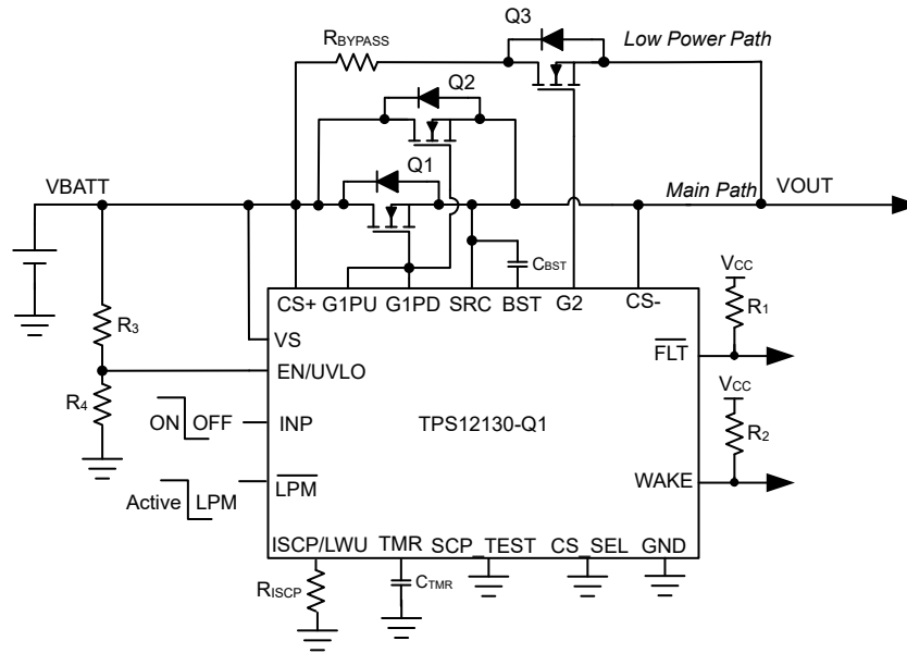
图 8-1. 适用于使用自动负载唤醒功能来驱动全时供电 (PAAT) 负载的 TPS12130-Q1 应用电路
