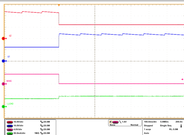
图 8-3. 从 LPM 到工作模式的状态转换 (LPM = 低电平, VIN = 12V, EN/UVLO = 高电平)
