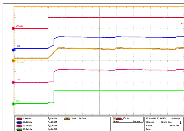
图 8-2. 低功耗路径的启动曲线 ( \overline{\text{LPM}} = 低电平, V_{\text{IN}} = 12\text{V} , 无负载, \text{CBST} = 470\text{nF} )
