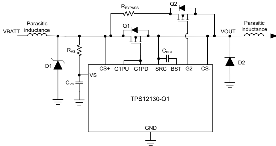
图 8-16. 采用可选保护元件的 TPS12130-Q1 电路实施方案
