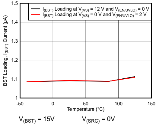
图 5-5. BST 负载电流 ( I_{(BST)} ) 与温度间的关系
