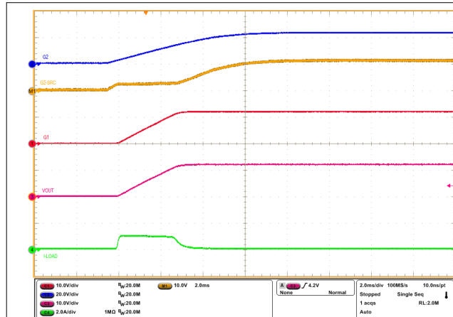
图 8-13. 输出端为 220 \mu F 时的浪涌电流曲线 (LPM = 低电平)
