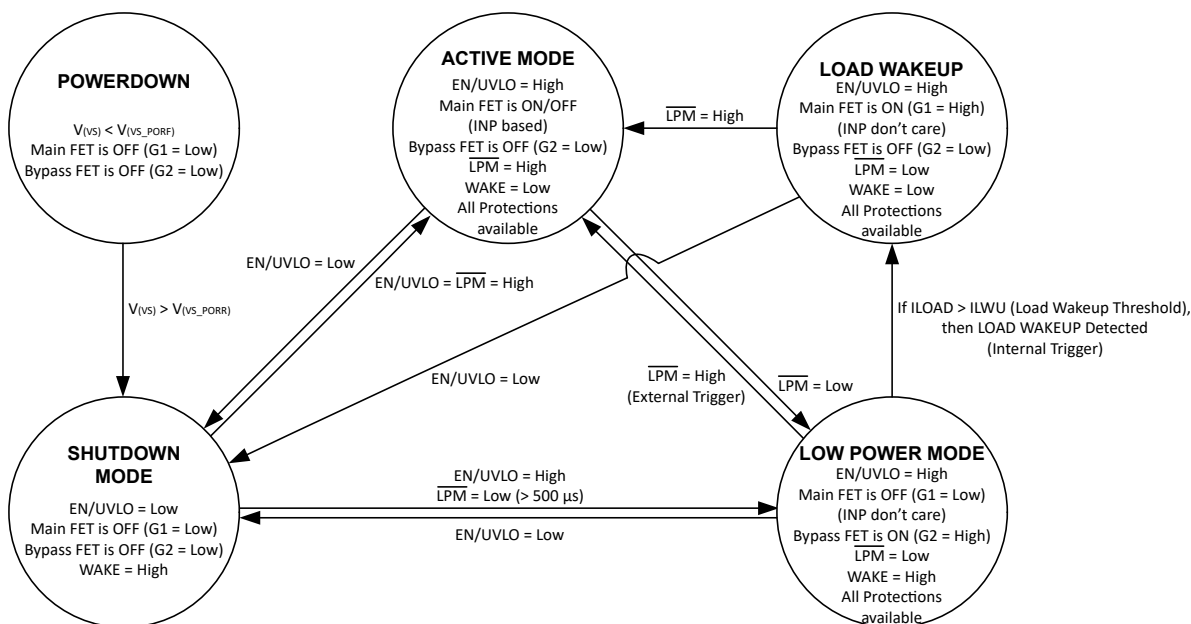
图 7-12. TPS12130-Q1 状态图
