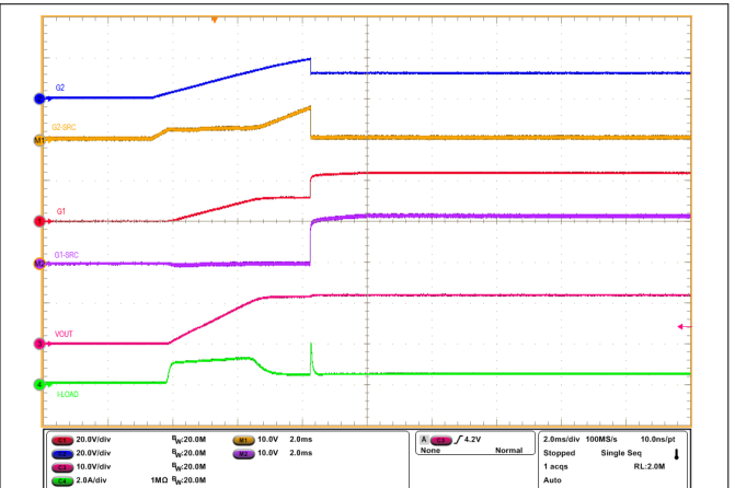
图 8-14. 输出端为 220 \mu F 且负载为 0.5A 时的浪涌电流曲线 (LPM = 低电平)
