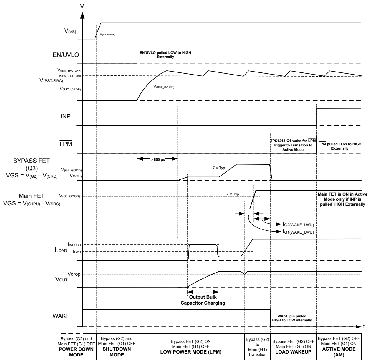
图 7-13. 包含负载唤醒事件的状态转换时序图
