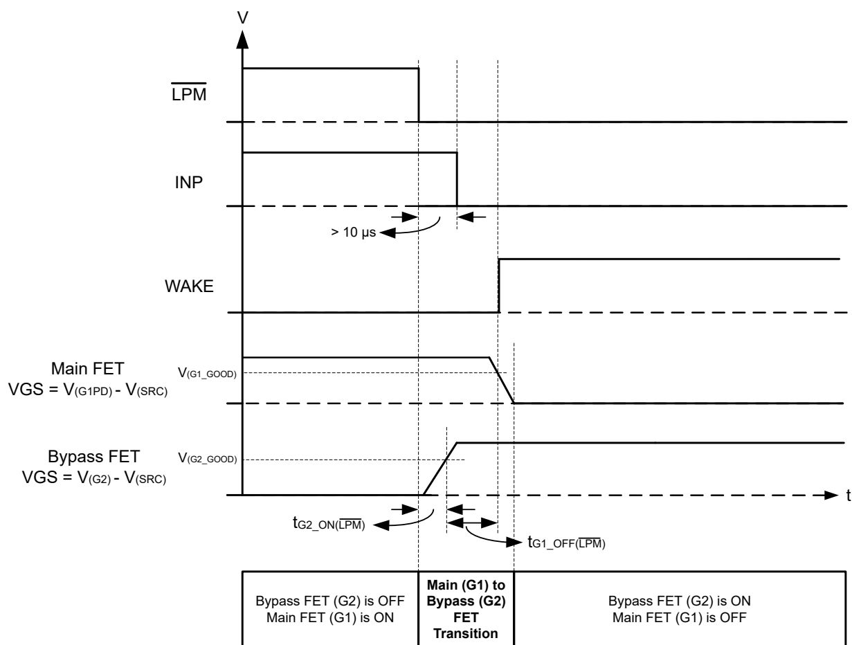
图 6-2. 通过 \overline{\text{LPM}} 触发器将工作模式转换为低功耗模式
