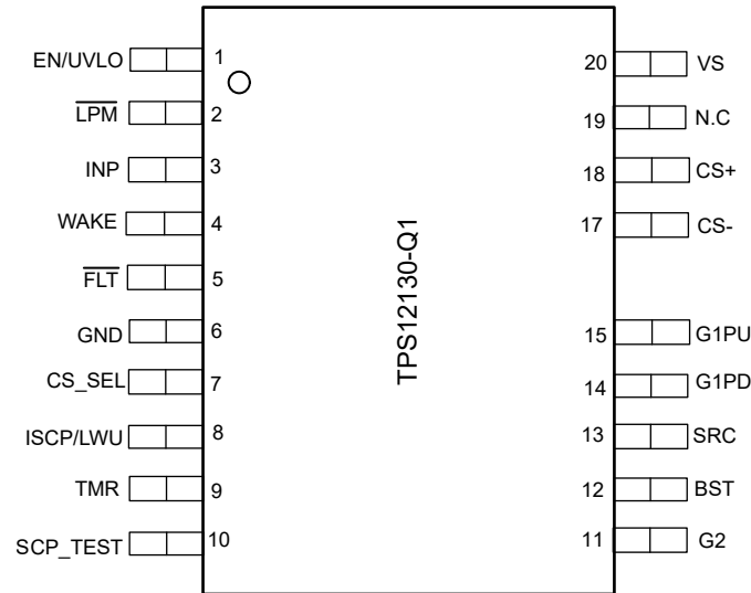
图 4-1. DGX 封装，19 引脚 VSSOP ( 顶视图 )
