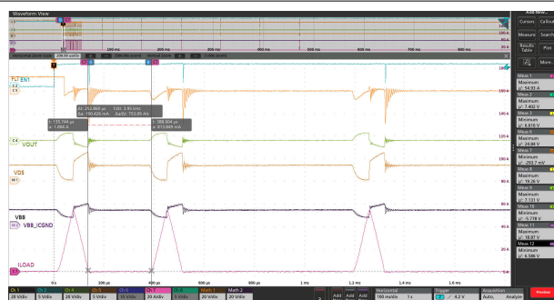
图 9-7. 上升压摆率 (P、M 版本)
