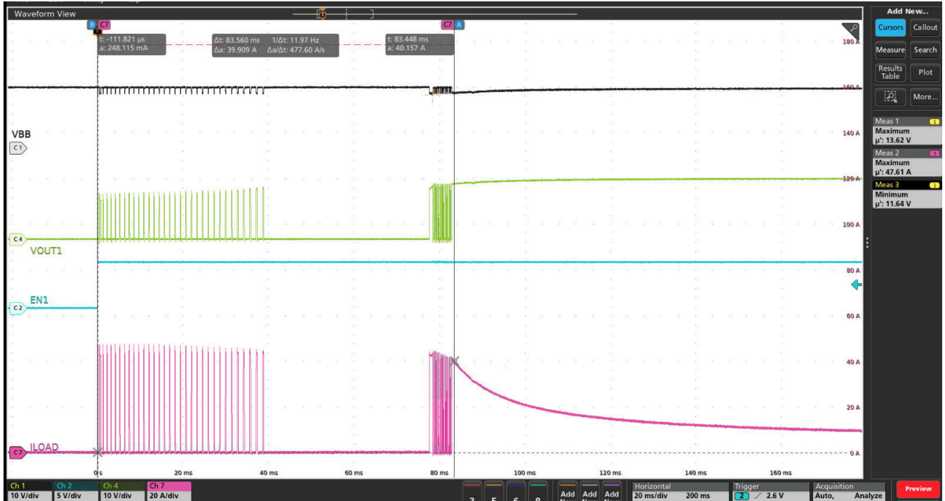
图 8-34. 使用 TPS1HC04-Q1 单通道在 13.5V VBB 下进行 100W 灯泡充电 ( T_A (device) = 25°C, T_A (bulb) = -40°C, ILIM = GND)
