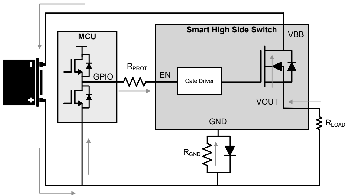
图 8-37. 电池反向电路
