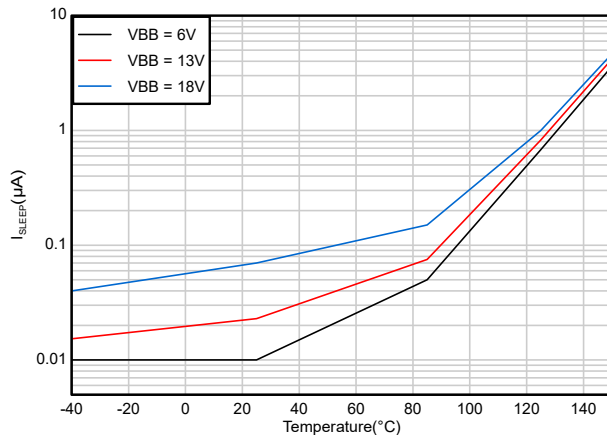
图 6-1. 待机电流 ( I_{SLEEP} ) 与温度间的关系
