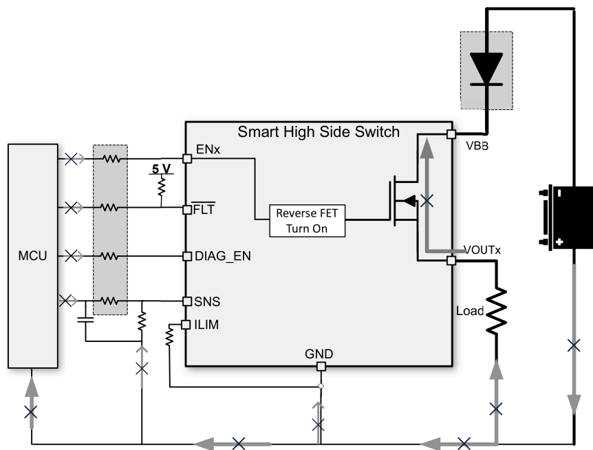
图 8-41. 采用阻断二极管实现反向保护
