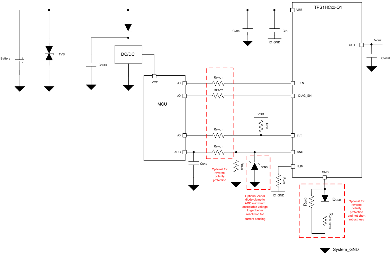
图 9-1. 典型应用图
