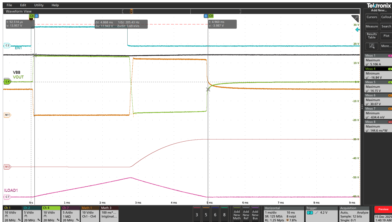
图 8-25. 5mH 电感负载驱动 ( V_{BB} = 13.5V , T_{AMB} = 125^{\circ}C )
