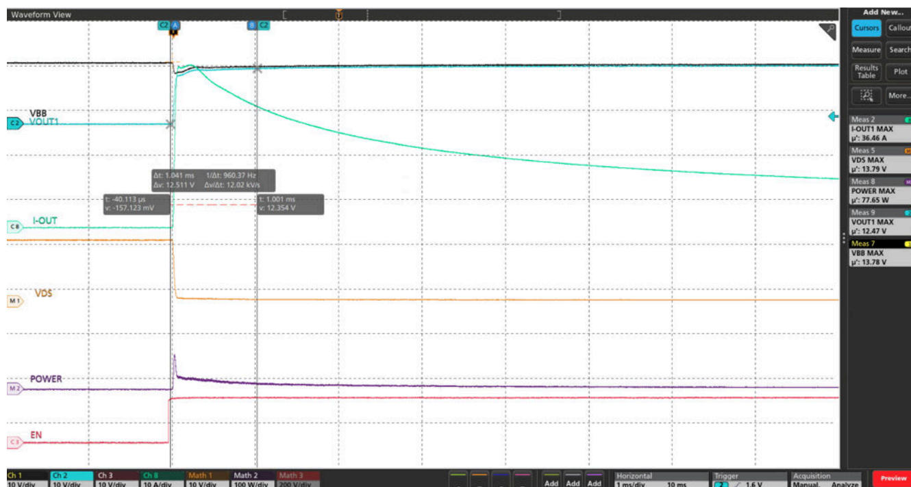
图 8-33. 使用 TPS1HC04-Q1 单通道在 13.5V VBB 下进行 35W 灯泡充电 ( T_A(\text{device}) = 25^\circ\text{C} , T_A(\text{bulb}) = -40^\circ\text{C} , ILIM = \text{GND} )
