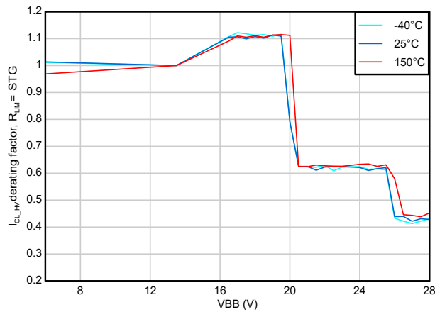
图 6-21. 电流限制降额因子 ( I_{CL\_HV} ) 与 V_{BB} 间的关系, R_{LIM} = STG
