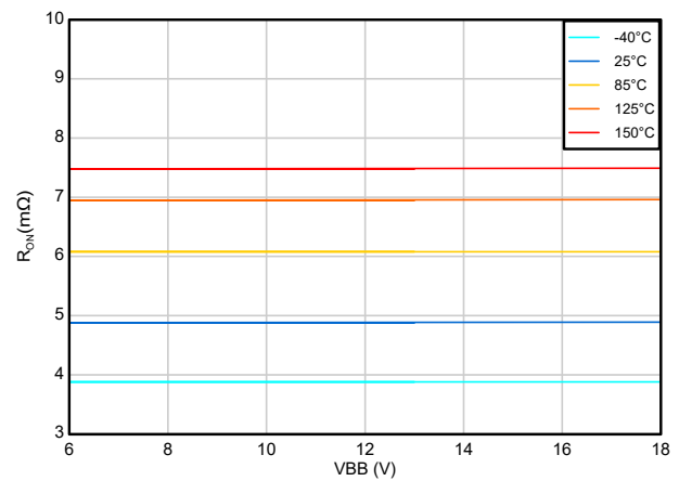
图 6-4. 导通电阻 ( R_{ON} ) 与 VBB 间的关系
