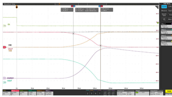
图 9-8. 下降压摆率 (P、M 版本)
