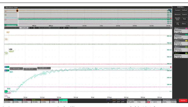
图 8-10. SNS 引脚带 150pF C_{SNS} 时的纹波 ( V_{BB} = 13.5V , I_{LIM} = \text{开路} , R_L = 10\Omega , R_{SNS} = 1k\Omega , T_A = 25^\circ C )
