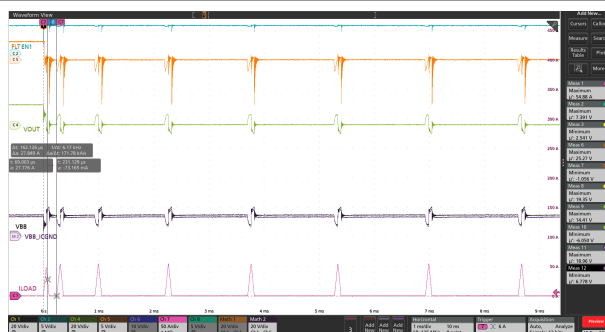
图 9-10. 器件上具有开路负载故障时的开路负载检测延迟 (P、D 版本)
