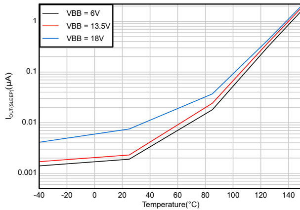
图 6-3. 输出泄漏电流 ( I_{OUT(SLEEP)} ) 与温度之间的关系
