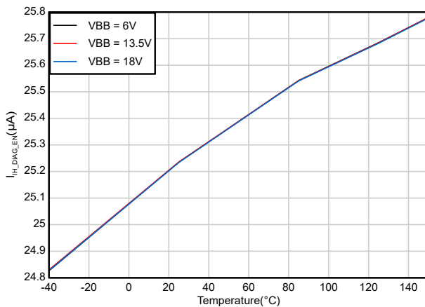
图 6-17. DIAG_EN 输入电流高电平与温度间的关系
