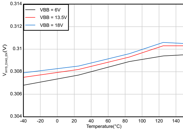
图 6-15. DIAG_EN 输入电压迟滞与温度间的关系
