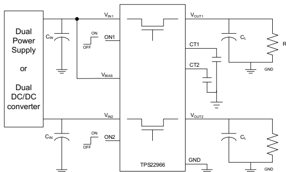
图 1. 典型应用
